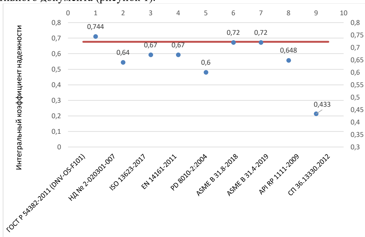
Рисунок 1 – Значения интегральных коэффициентов надежности
