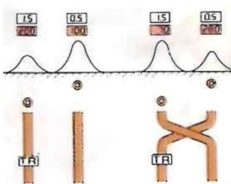
Рисунок 2 – Возможные расположения на местности труб и кабелей электропитания
