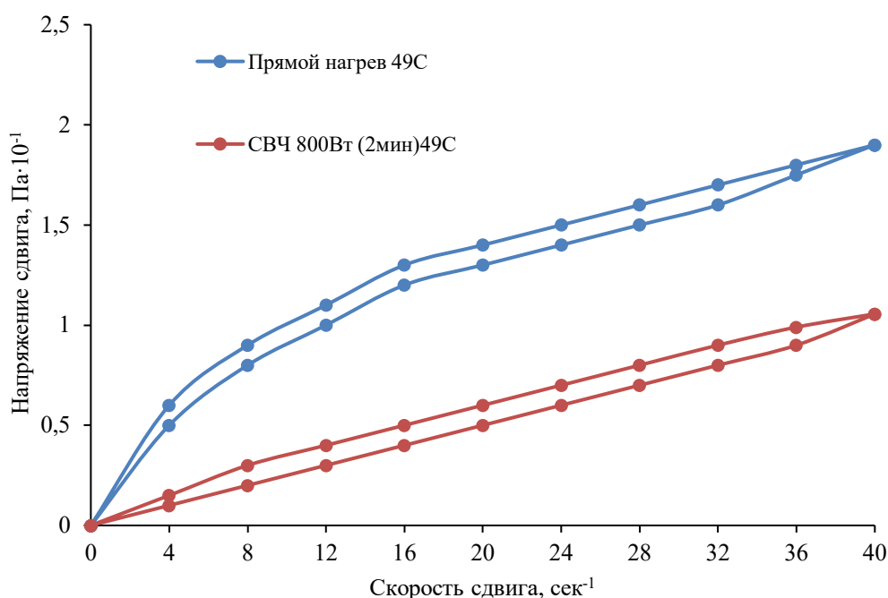
Рисунок 1 – Кривая течения образца тяжелой нефти
