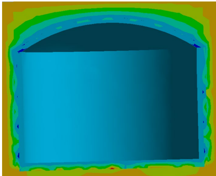
Рисунок 2 – Результаты расчета и графическое отображение теплообмена ИР с окружающей средой
