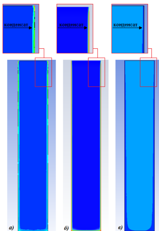
а – модель Wet Steam, б – модель Volume of fluid (VOF), в – модель Mixture
