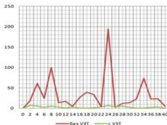
Рисунок 2 – Плотность тока утечки на участке сближения ВЛ и трубопровода после установки УЗТ
