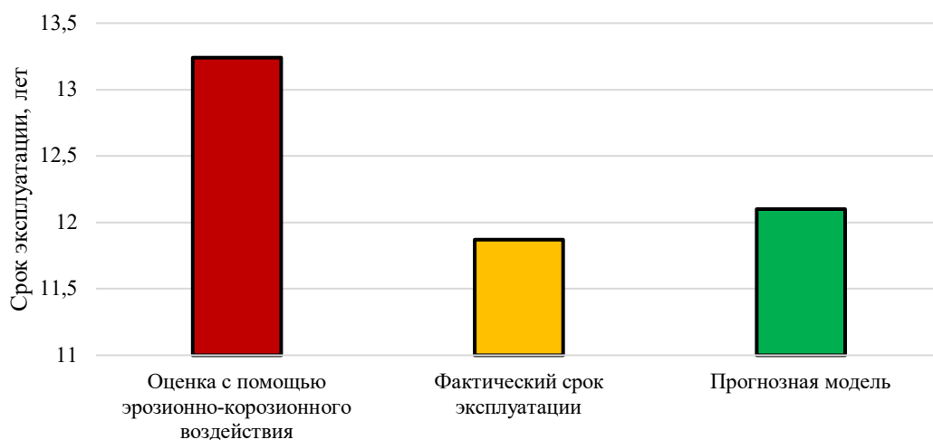
Рисунок 2 – Сравнение методов расчета остаточного ресурса трубопроводов
