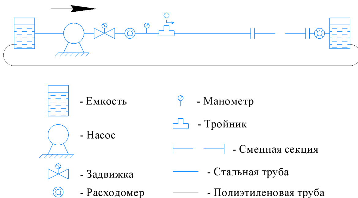
Рисунок 1 – Принципиальная схема экспериментального стенда
