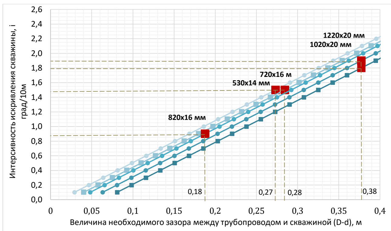
Рисунок 1 - Номограмма предельной интенсивности искривления скважины
