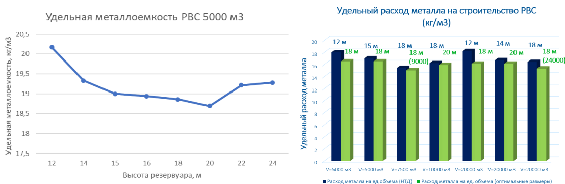
Рисунок 1 – Удельный расход металла на сооружение РВС-5000 и сравнительный анализ удельного расхода металла на сооружение РВС для разных диаметров и высот конструкции
