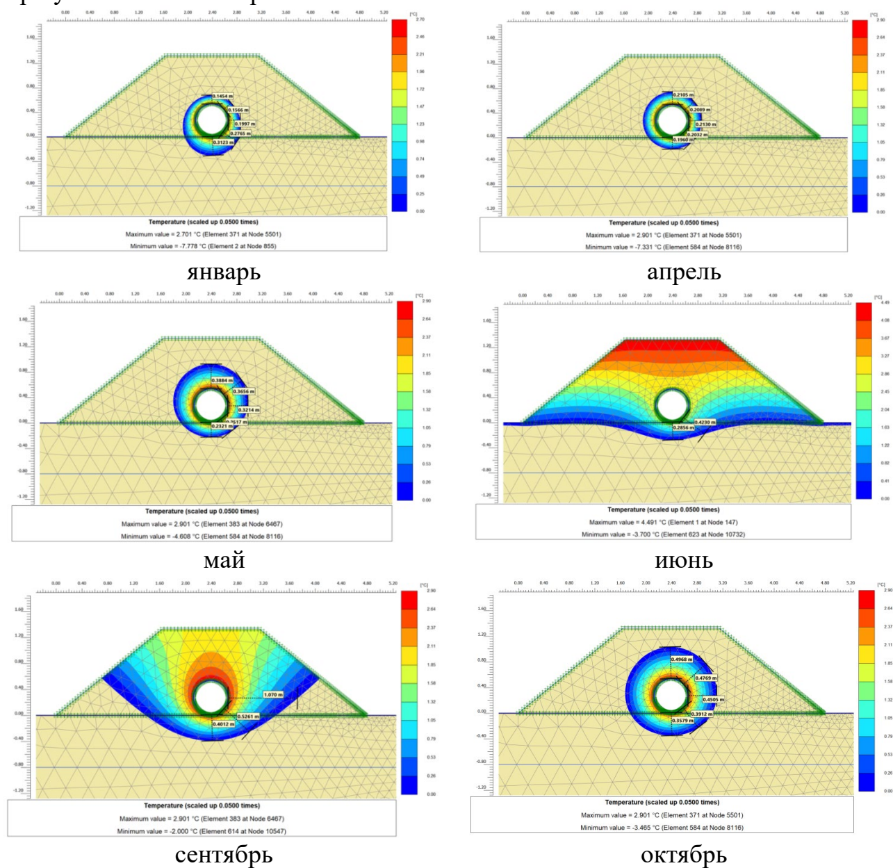
Рисунок 1 – Изолинии температуры по месяцам в годовом цикле регулирования теплообмена трубопровода с окружающей средой
