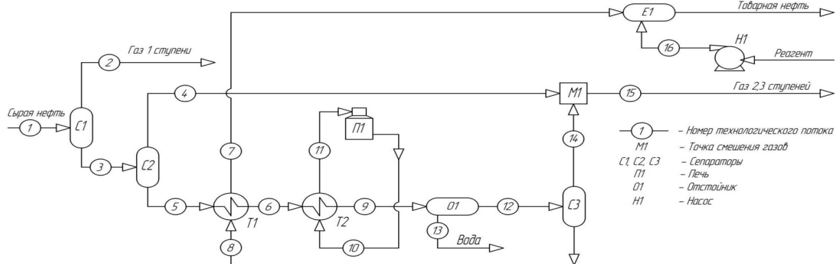
Рисунок 1 – Схема технологического процесса подготовки нефти
