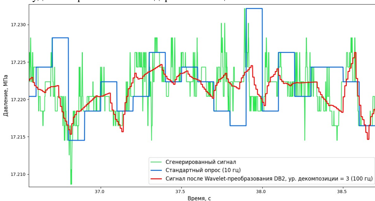
Рисунок 1 – Сравнение полученных сигналов
