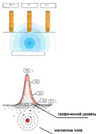
Рисунок 1 – Магнитное поле рассеивания вблизи одиночной подземной металлической трубы
