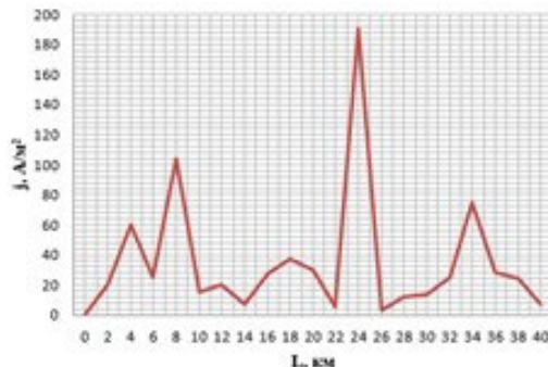
Рисунок 1 – Плотность тока утечки с возможных дефектов в защитном покрытии газопровода-отвода на участке сближения
