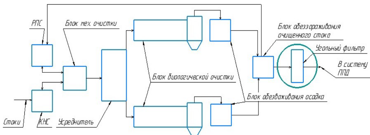
Рисунок 1 – Схема канализационных очистных сооружений (КОС)
