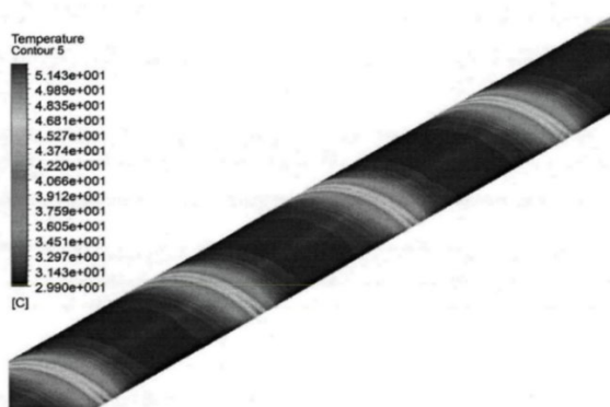
Рисунок 2 – Температурное поле на стенке трубы при спиральном расположении нагревательного элемента
