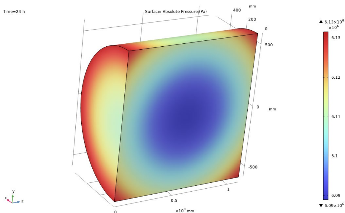
Рисунок 2 – Распределение давления через 24 часа после начала процесса охлаждения
