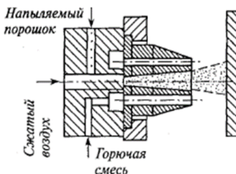
Рисунок 2 - Схема воздушно-пламенного напыления
