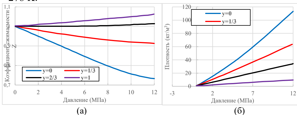
Рисунок 1 – Влияние различного содержания водорода «у» в смеси водорода с природным газом при изотермическом режиме: (а) коэффициента Z (б) плотности, при различных давлениях и температуры ( T = 278 К)
