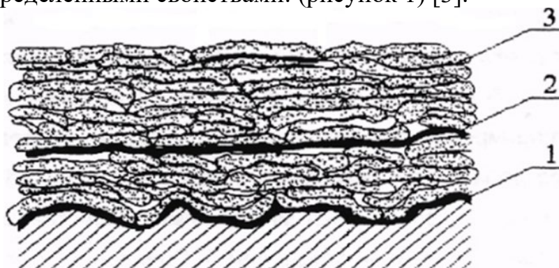
Рисунок 1 – Схема структуры напыленного покрытия
