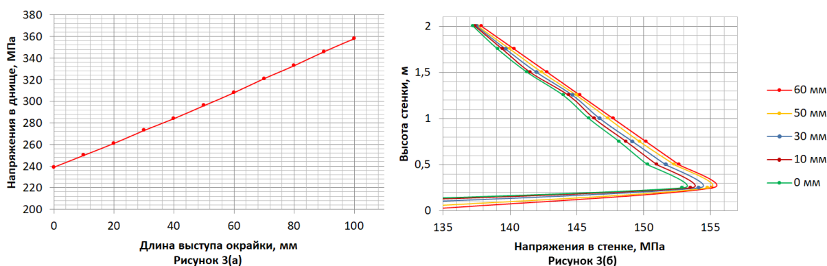
Рисунок 2 – Напряжения в уторном узле на примере конструкции РВСП-50000 с различными выступами кольцевых окрайек, возникающие в днище и резервуара
