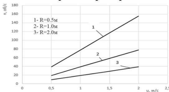
Рисунок 2 - Зависимость n=f(u)
