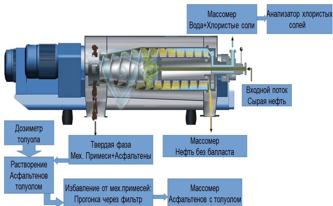
Рисунок 1 – Блок-схема САОСБН на основе трёхфазной центрифуги (трикантера)
