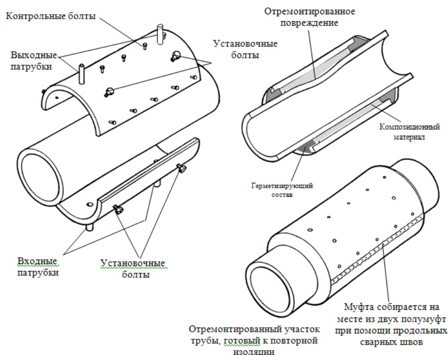
Рисунок 1 – Схема установки композитно-муфтовой ремонтной конструкции
