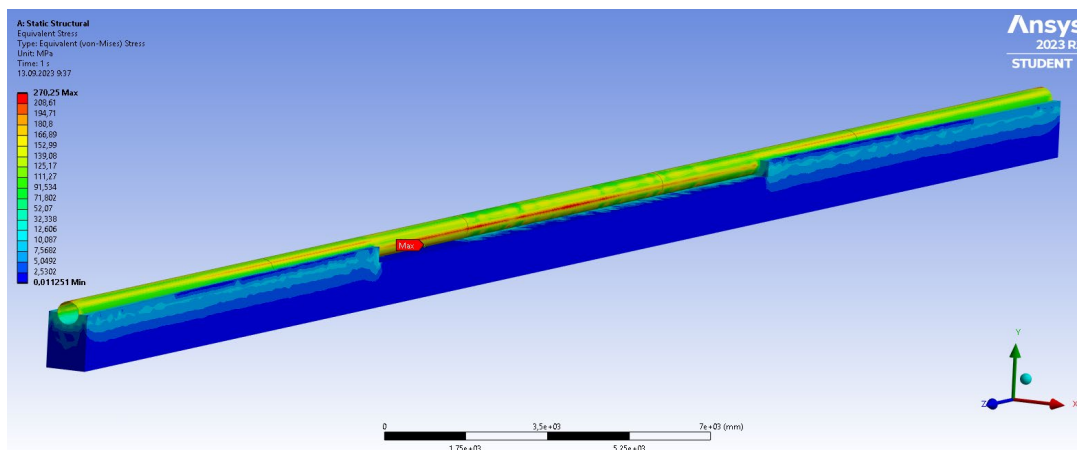
Рисунок 3 – График распределения напряжений после применения криогеля (max = 270,25 МПа)
