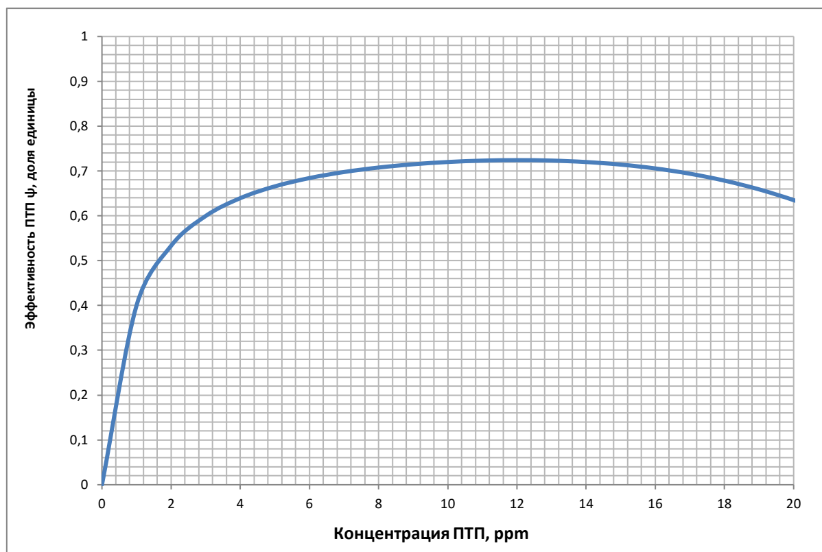
Рисунок 1 – Математическая модель зависимости гидравлической эффективности присадки от концентрации ПТП
