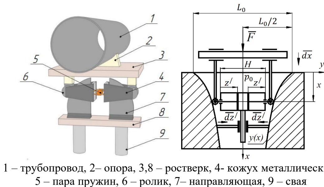
Рисунок 1 – Конструкция сейсмозащиты на пружинах (слева), на пневмопружинах (справа)
