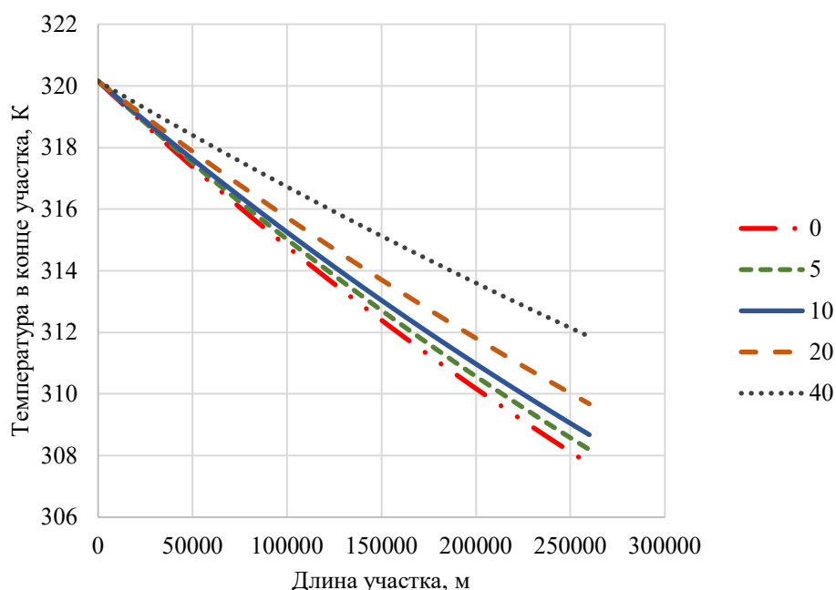
Рисунок 2 – Зависимость температуры в конце участка от длины при различных значениях гидравлической эффективности ПТП
