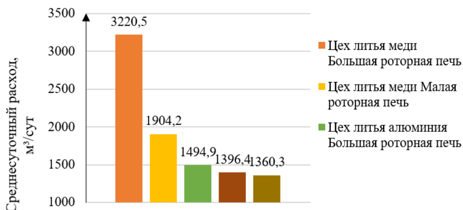
Рисунок 1 – Расходы топливного газа по печам
