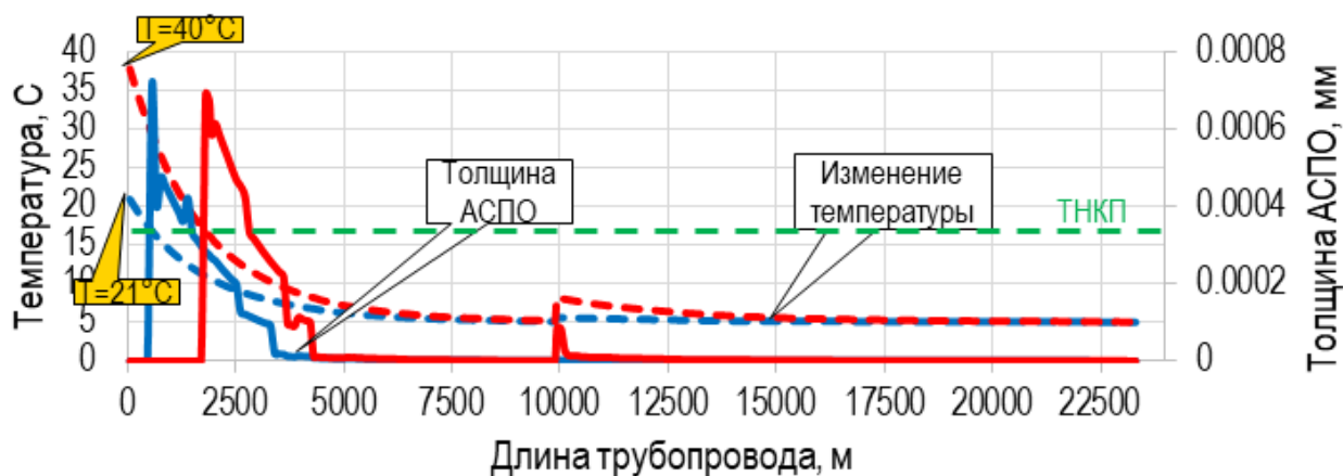
Рисунок 2 – Результат гидравлического расчета трубопровода для наглядного определения участков образований АСПО в зимний период
