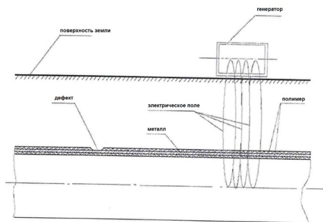
Рисунок 3 – Схематическое представление активизации магнитного поля рассеяния с помощью катушки индуктивной связи
