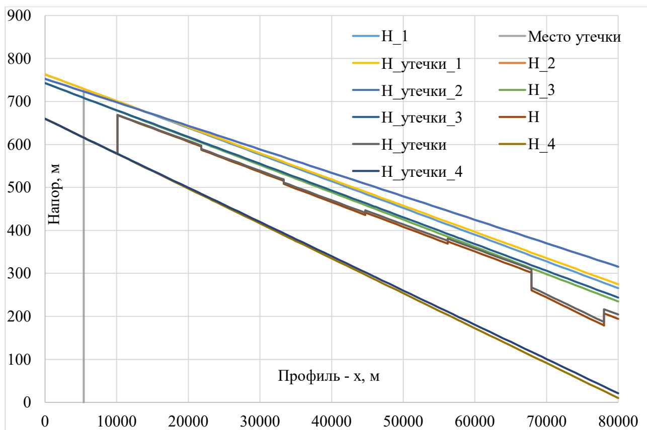
Рисунок 1 – График напора для перекачки нескольких продуктов при наличии и отсутствии утечки и общий график гидравлического уклона нефтепродуктопровода
