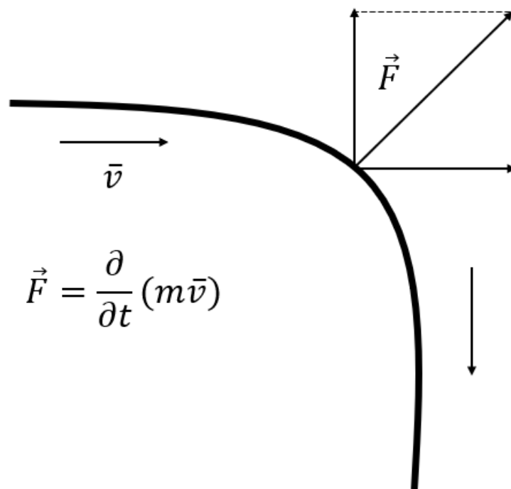
Рисунок 1 – Ударная сила при изменении направления жидкостной пробки
