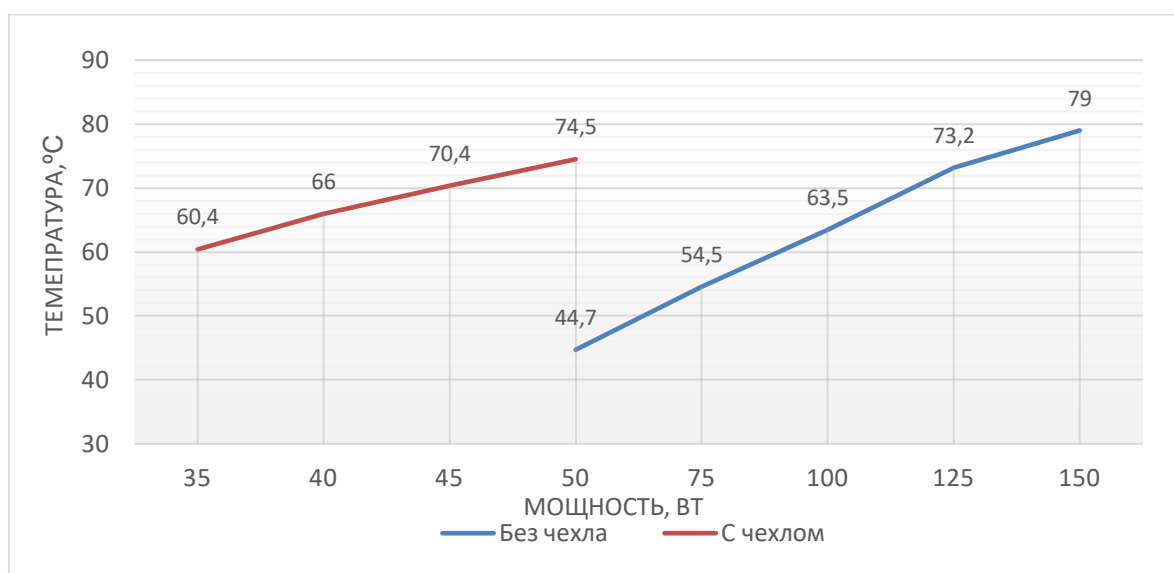
Рисунок 2 – Зависимости температуры воды от мощности нагревателя без использования и с использованием термочехла
