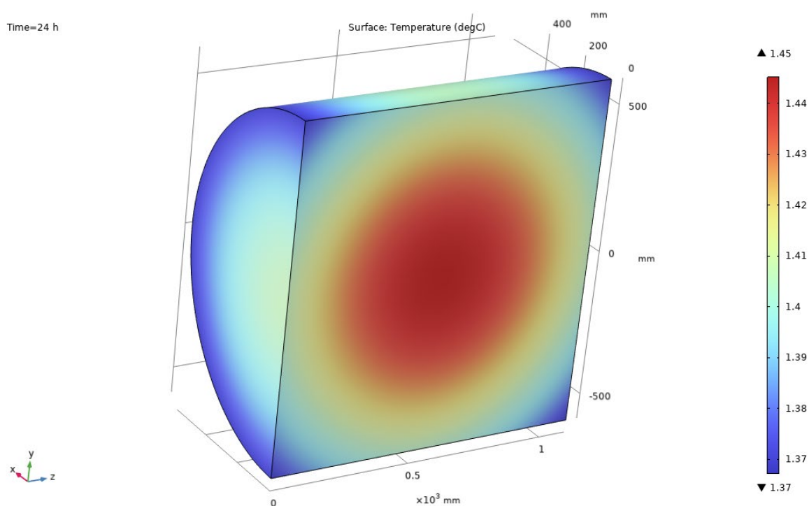
Рисунок 1 – Распределение температуры через 24 часа после начала процесса охлаждения
