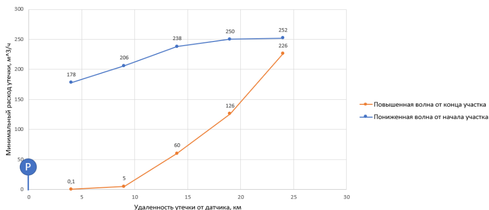
Рисунок 3 – Объем минимально возможной обнаруживаемой утечки
