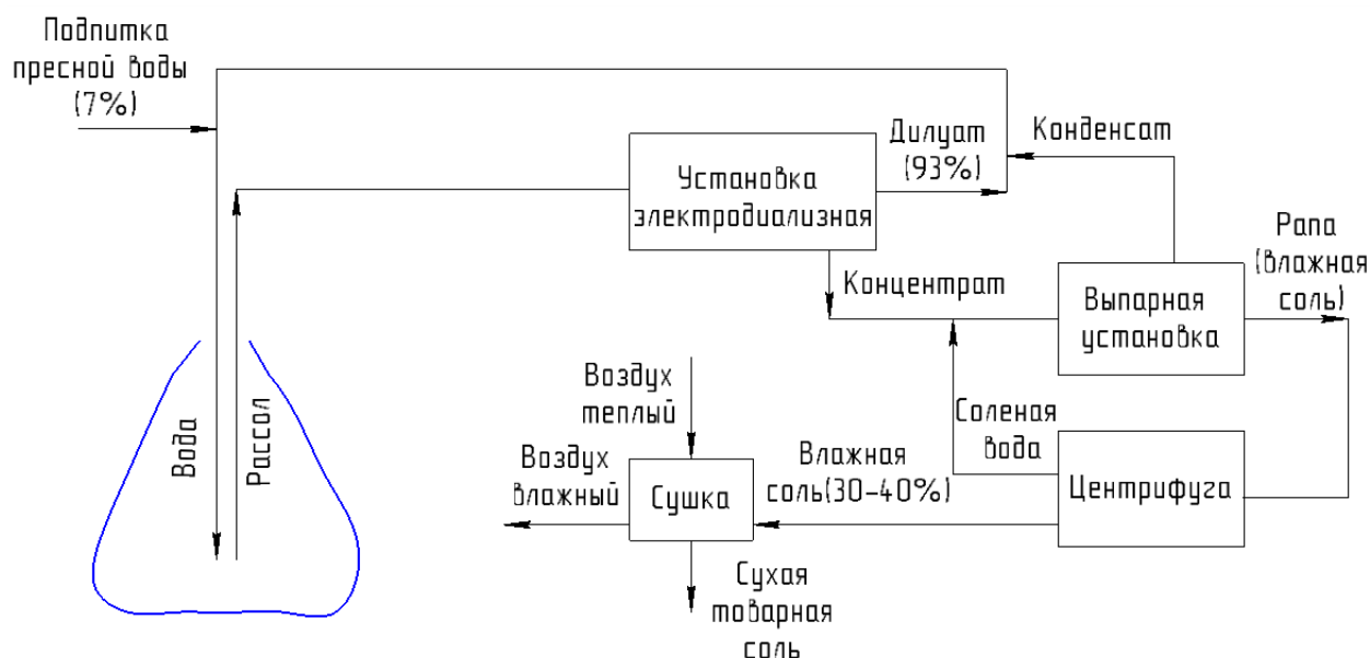
Рисунок 2 – Технологическая схема замкнутого водооборотного цикла при создании полости в пластах каменной соли
