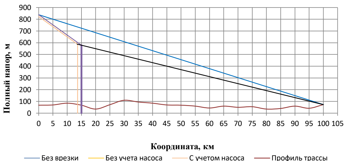
Рисунок 1 – Определение координаты врезки, совершенной на 15 км, при откачке 5%
