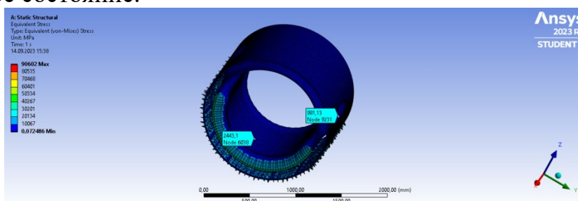
Рисунок 2 – Распределение напряжений в системе «футляр-компенсатор-труба»
