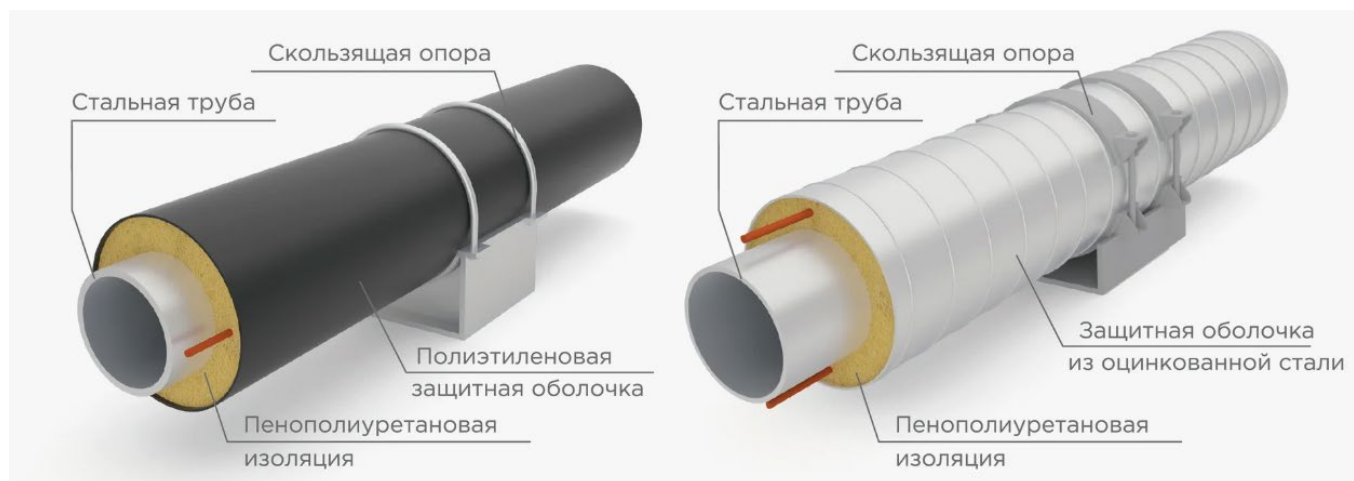
Рисунок 1 – Трубы в ППУ изоляции с разными защитными оболочками
