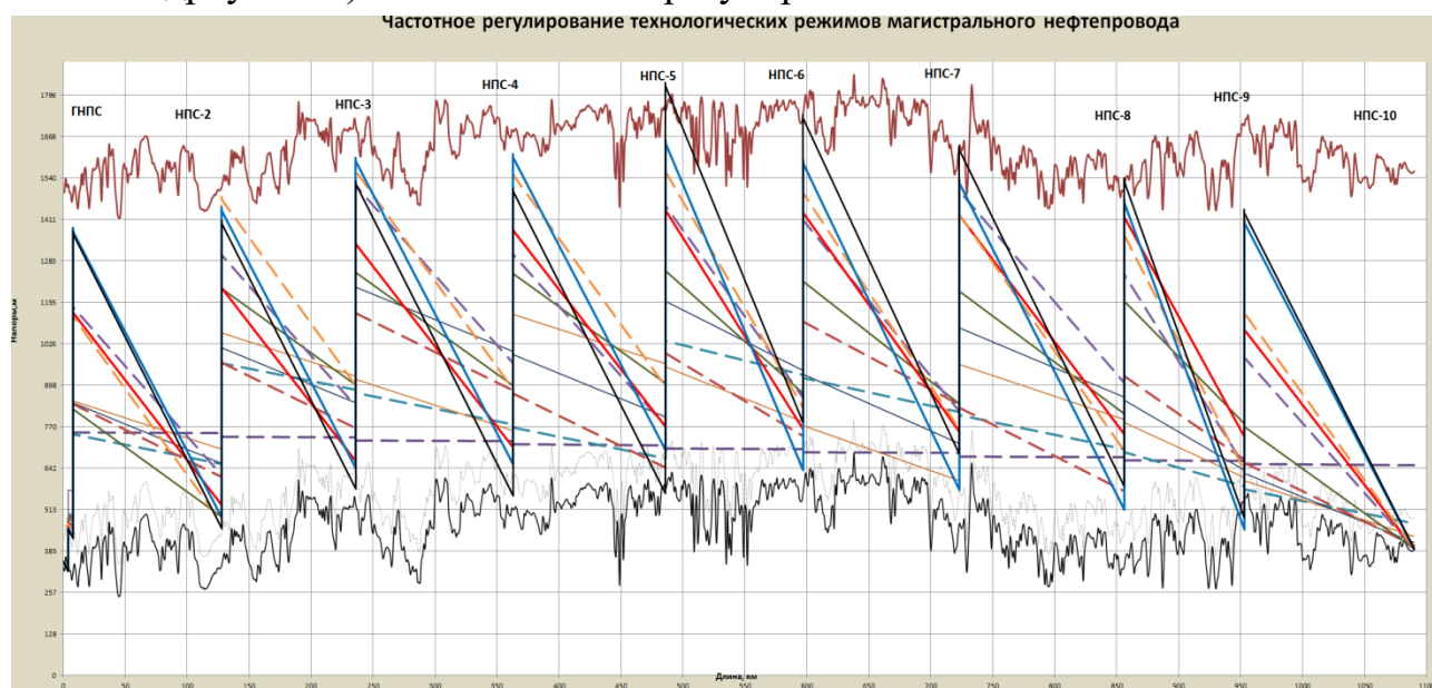
Рисунок 1 - Линии гидроуклонов технологического участка
