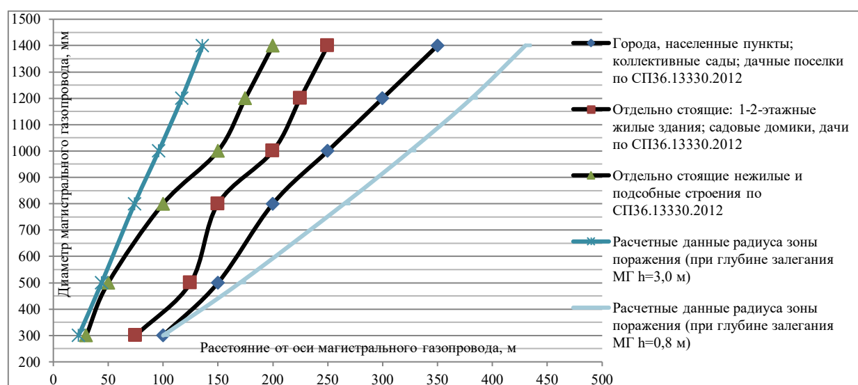
Рисунок 1 – Графическое отображение результатов анализа параметров зон поражения (разлет осколков) при глубине залегания МГ h=0,8 м и h=3,0 м (до верхней образующей трубы), а также сравнение со значениями ЗМР по таблице 4 [4]
