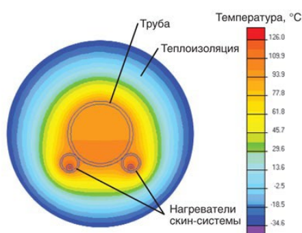
Рисунок 1 – Температурное поле при наличии двух нагревательных элементов
