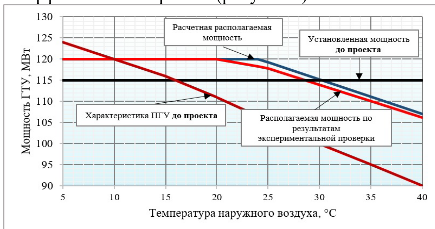
Рисунок 1 – Сравнение результатов расчетно-теоретических исследований и экспериментальной проверки
