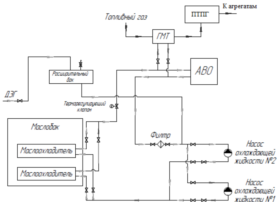
Рисунок 1 – Принципиальная схема внедрения ГМТ в систему охлаждения ДЭГ
