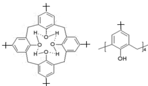
Рисунок 1 Структура каликс[4]арена, продукта циклической олигоконденсации четырёх молекул p -трет-бутилфенола и четырёх молекул формальдегида
