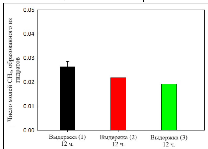
Рисунок 2 – Результаты молей \text{CH}_4 , образующегося из газогидратов во время каждой выдержки
