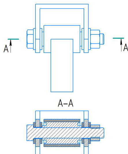
Рисунок 2 – Сайлентблок
