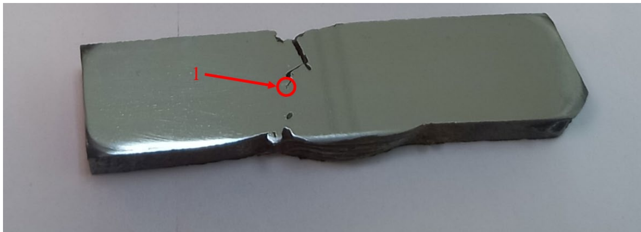
Рисунок 1 – Вырезанный образец из фрагмента газопровода
