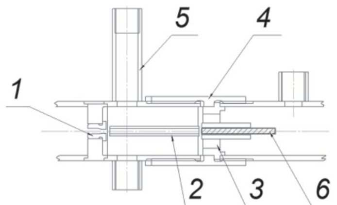
1 – сменное сопло; 2 – сменный резонатор; 3 – сменное основание резонатора; 4 – муфта резьбовая; 5 – патрубки для датчиков; 6 – термопара концевая Рисунок 2 – Конструкция экспериментальной установки
