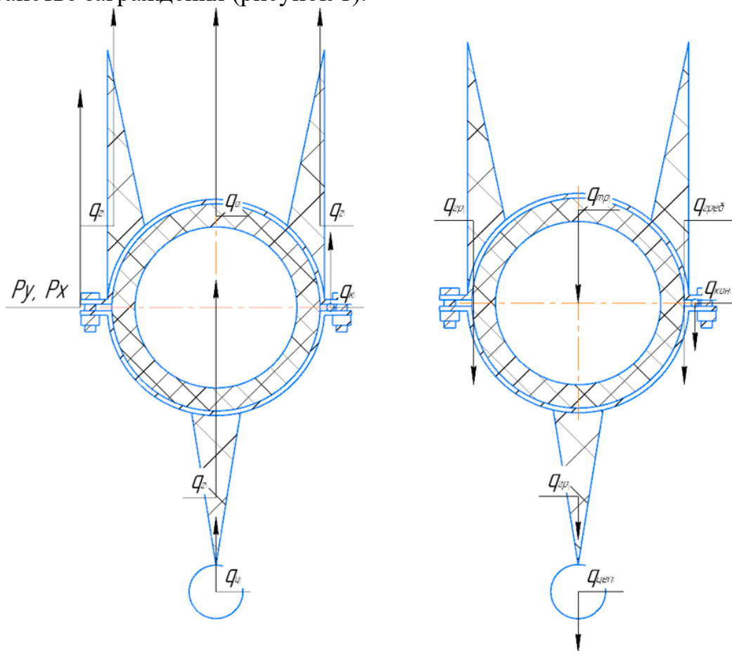
Рисунок 1 – Активные и пассивные нагрузки, действующие на заграждение
