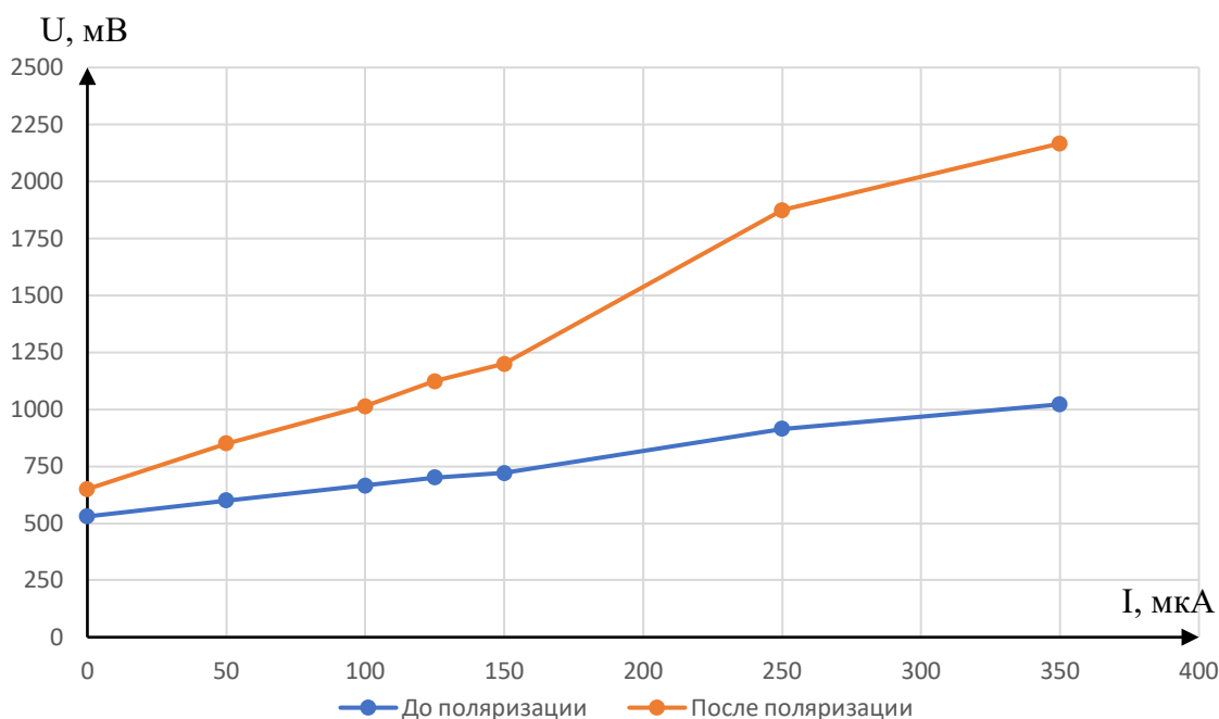
Рисунок 2 – Поляризационные кривые образца до и после катодной поляризации током высокой плотности
