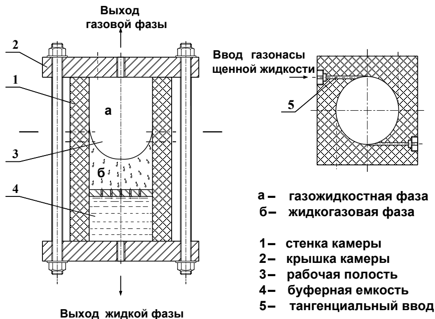
Рисунок 1 – Вихревая камера
