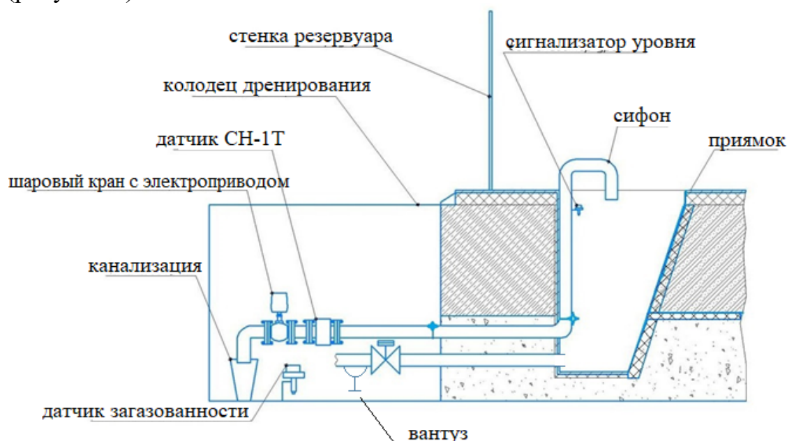
Рисунок 1 - Конструктивное исполнение предлагаемой системы
