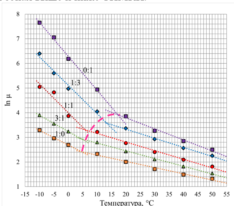
Рисунок 1 – Определение ТНМКП в бинарной смеси при различных концентрациях исходных смешиваемых нефтей
