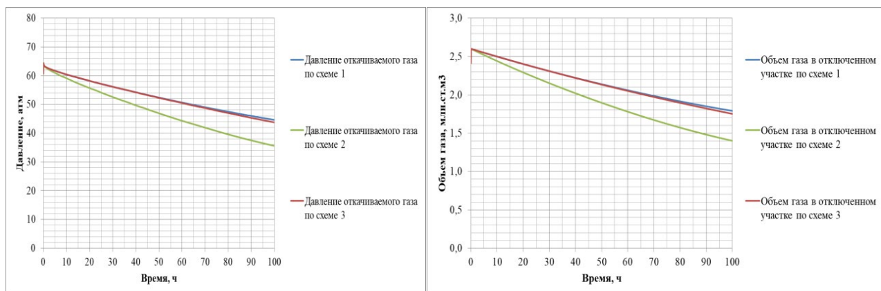
Рисунок 1 – Давление и объем технологического газа, остающегося в отключенном участке
