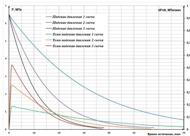
Рисунок 1 – Графики изменения давления и темпа падения давления во времени
