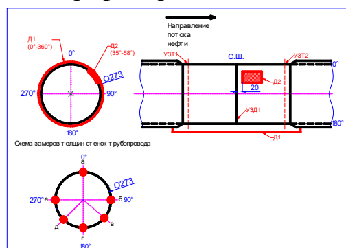
Рисунок 2 – Схема расположения дефекта при ДДК №2
