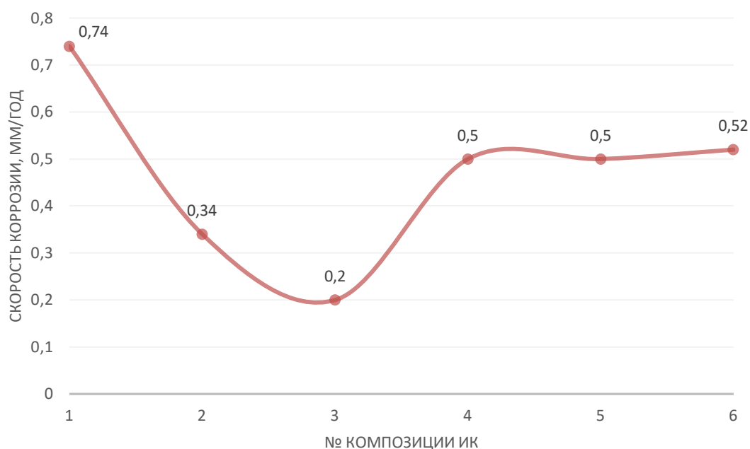
Рисунок 2 – Зависимость скорости коррозии от концентрации добавки K_2Cr_2O_7
