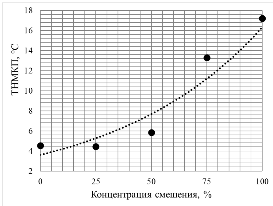
Рисунок 2 – Характер поведения ТНМКП в бинарной смеси нефтей в зависимости от концентрации смешения
