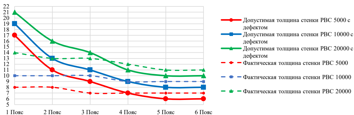
Рисунок 1 – Дефект с высотой 1500 мм
