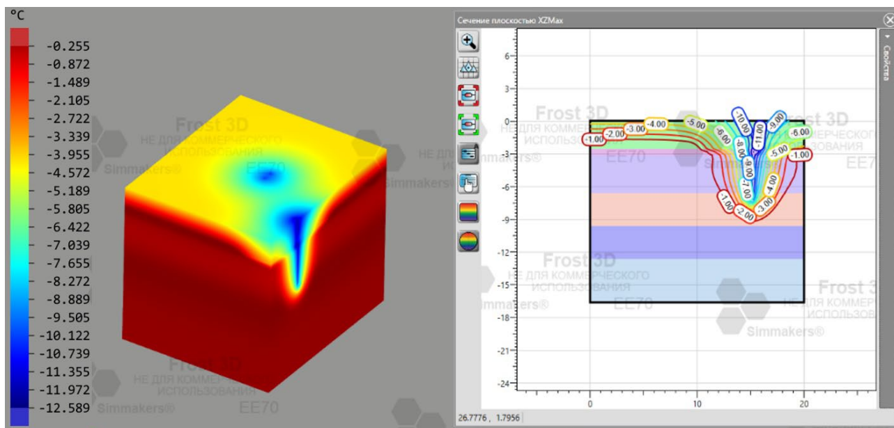
Рисунок 1 – Моделирование теплового взаимодействия опор трубопроводов с установленными термостабилизаторами с многолетнемерзлым грунтом Основания в программном комплексе Frost 3D
