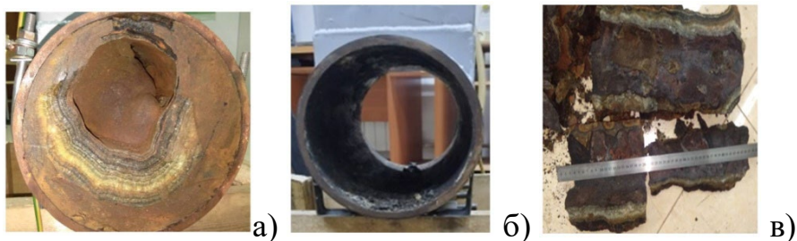
Рисунок 1 – Лабораторные испытания установки ЭГДУ-ТО с удалением ТСО (гипсы)+АСПО на отрезке нефтепровода Ø219 мм: а – отрезок нефтепровода с закупоркой сечения трубы более 90%; б - отрезок трубы после удаления ТСО; в – фрагменты ТСО
