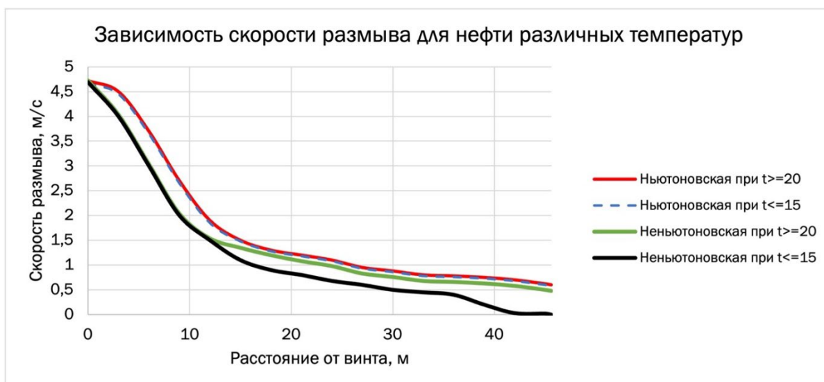
Рисунок 1 – Зависимость скорости размыва нефти в резервуаре для различных температур
