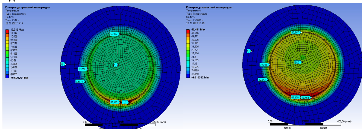
Рисунок 1 – Изменение температурного нефтепровода в результате расчета – 72 часа
