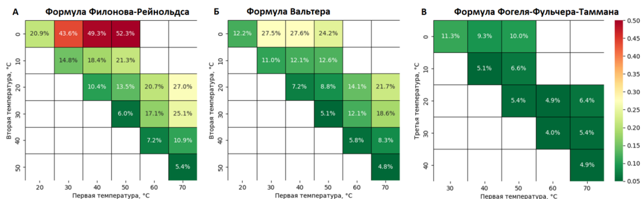
Рисунок 1 - Относительная погрешность при определении вязкости с помощью формул Филонова-Рейнольдса (А), Вальтера (Б), Фогеля-Фульчера-Таммана (В) при расчете внутри температурного диапазона
