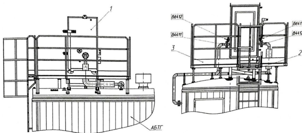
1 – газомасляный теплообменник; 2 – опора ГМТ; 3 – ограждение
