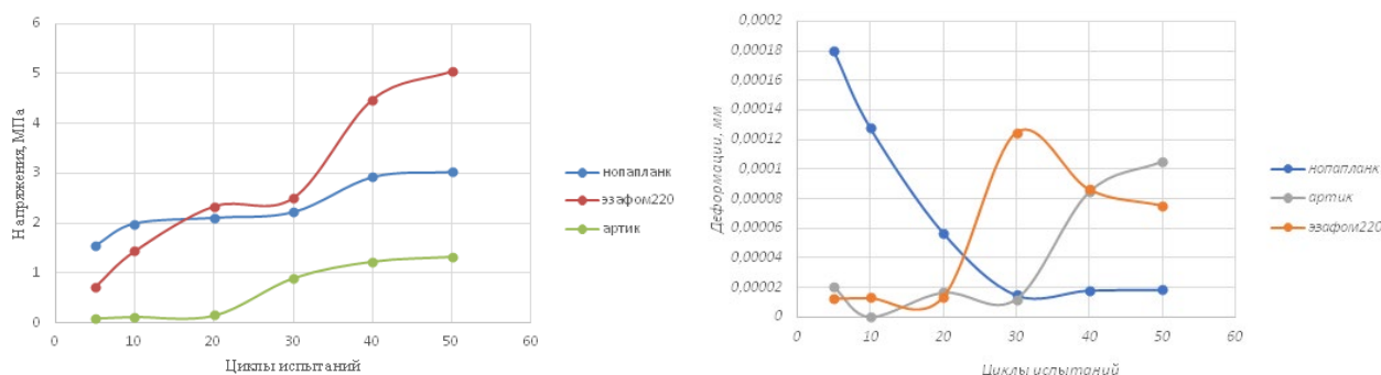
а) распределение напряжений б) распределение деформаций Рисунок 1 – Результаты численного моделирования распределений НДС в кожухе и трубе по числу циклов
