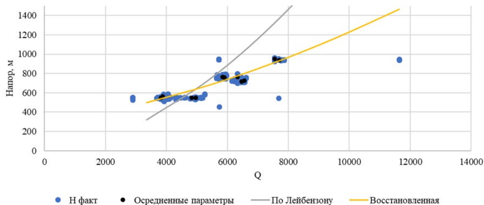
Рисунок 2 – Сопоставление теоретической гидравлической характеристики и фактических потерь энергии на трение
