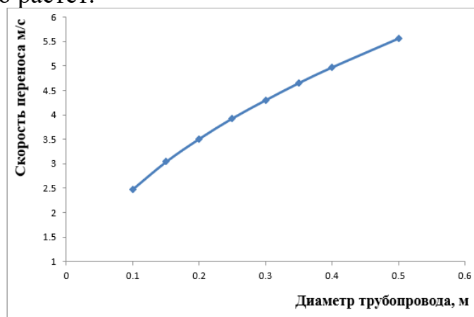
Рисунок 1 Зависимость скорость переноса механических частиц в газовом потоке для различных диаметров газопровода
