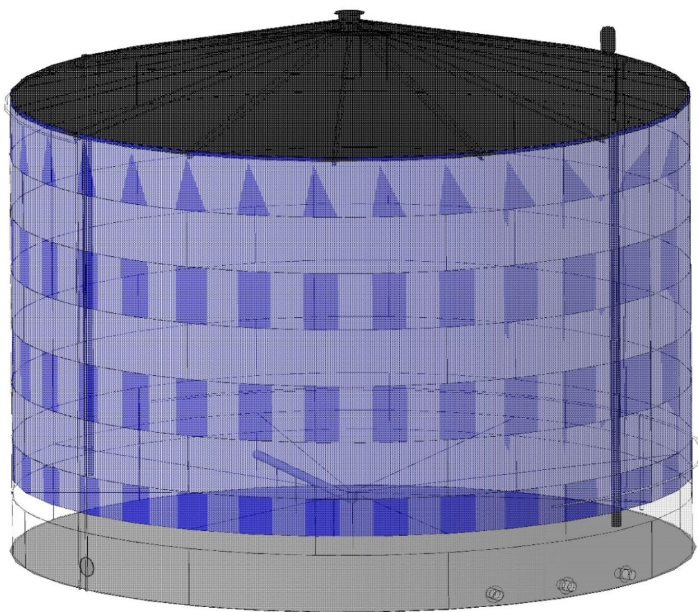
Рисунок 1 – Вид резервуара с мягкой оболочкой со стороны приемо-раздаточных патрубков
