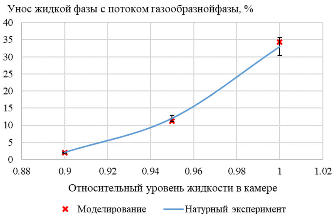
Рисунок 2 – Сравнение результатов натурных экспериментов и моделирования
