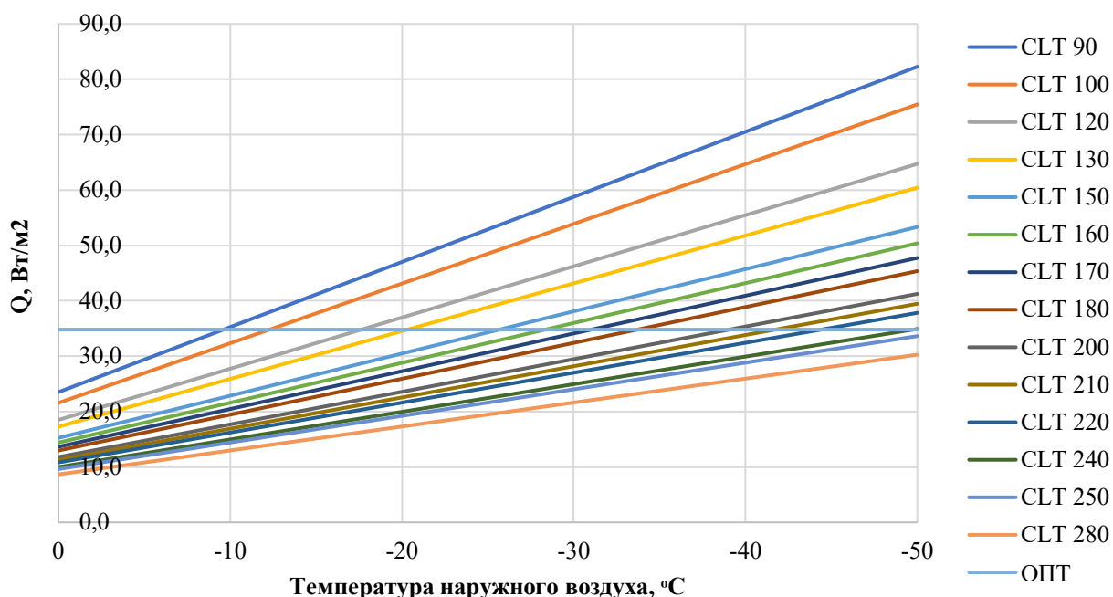
Рисунок 1 – График определения допустимой толщины CLT панелей при различных температурах наружного воздуха.
