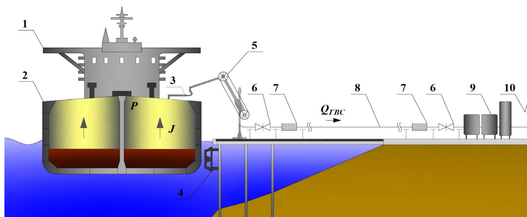
1 – танкер; 2 – двойной корпус; 3 – мастрейзер; 4 – узел защиты причальных сооружений; 5 – стендер отвода газовой фазы 6 – запорно-регулирующая арматура; 7 – детонационный преградитель; 8 – трубопровод отвода газовой фазы; 9 – установка рекуперации паров нефти; 10 – свеча рассеивания Рисунок 2 – Принципиальная схема процесса налива танкера
