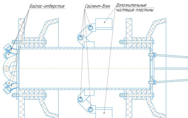
Рисунок 1 – Очистное устройство с дополнительными чистящими пластинами
