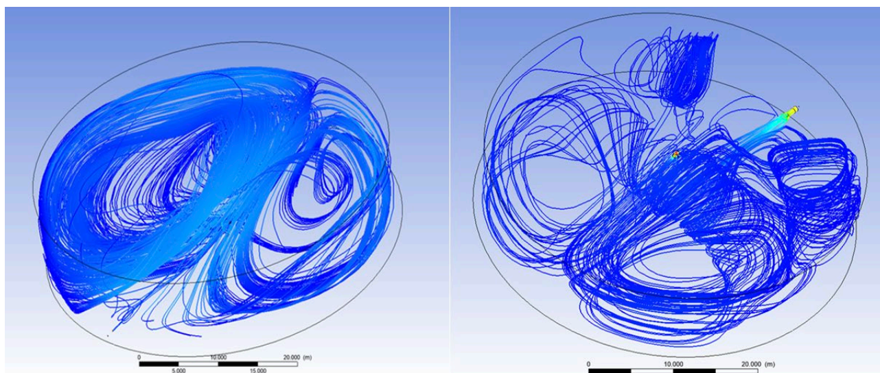
Рисунок 2 – Размыв донных отложений с использованием «УПС-ЕВНАТ» (слева) и с использованием «ДИОГЕН-700» (справа)
