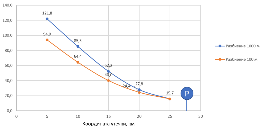
Рисунок 1 – Влияние расположения утечки на величину импульса в процентах от среднего давления на участке
