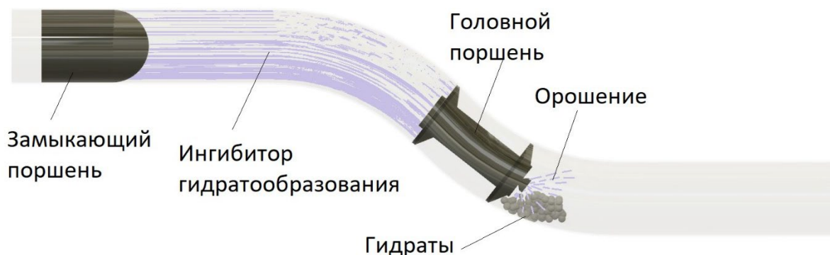
Рисунок 1 – Встреча головного поршня гидратной пробки
