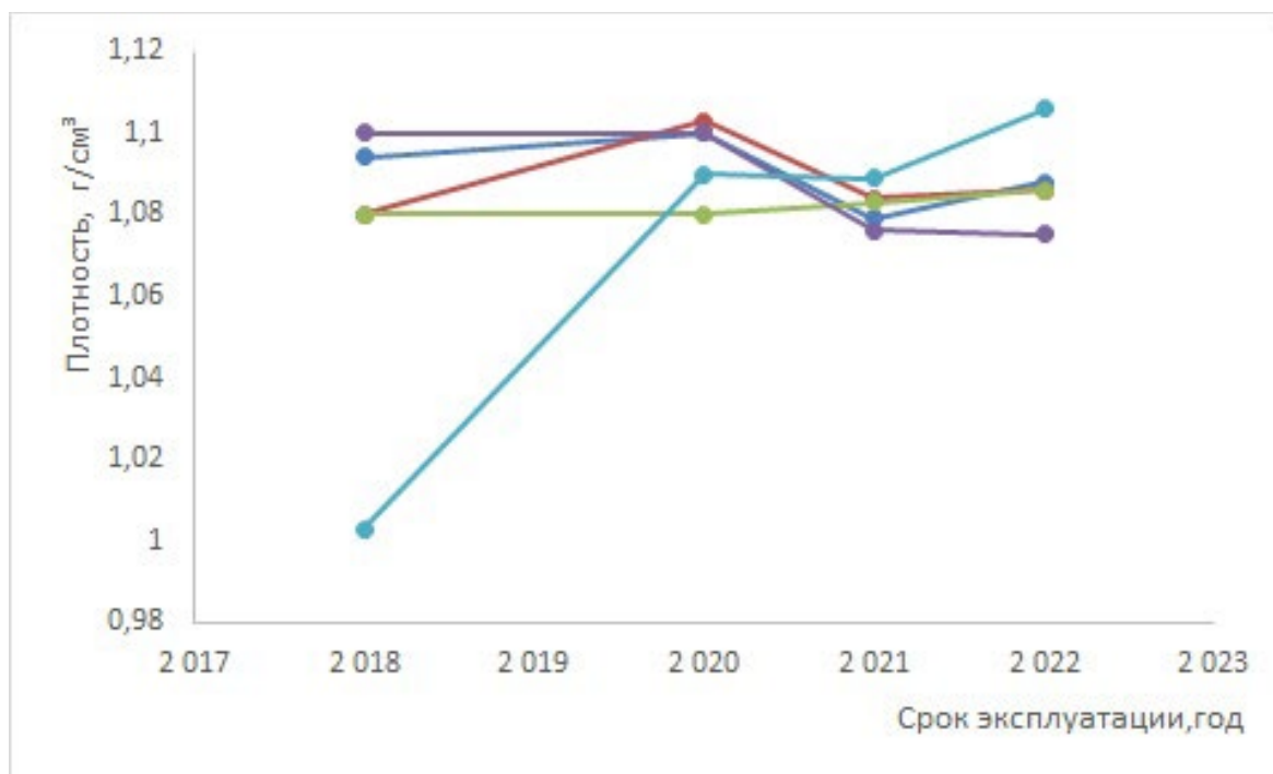
Рисунок 1 – Зависимость плотности проб промежуточного теплоносителя от срока эксплуатации подогревателей газа
