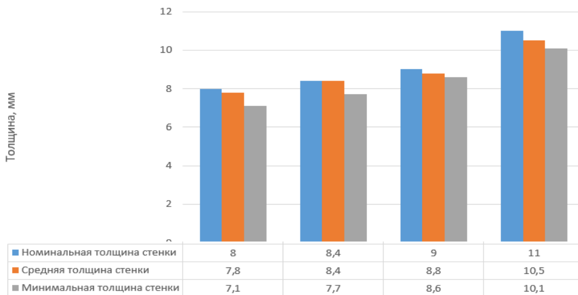
Рисунок 1 – Средняя и минимальная толщина стенки для выбранных номинальных толщин стенок
