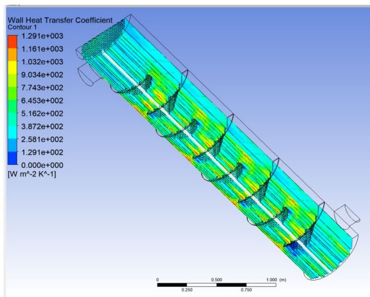
Рисунок 1 – Коэффициент теплоотдачи в теплообменнике с солевыми отложениями
