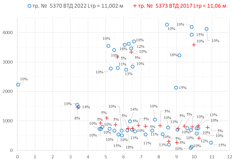
Рисунок 1 – Труба № 5373 ВТД 2017 года и труба № 5370 ВТД 2022 года магистрального газопровода «Новопсков-Аксай-Моздок» 127 – 0 км
