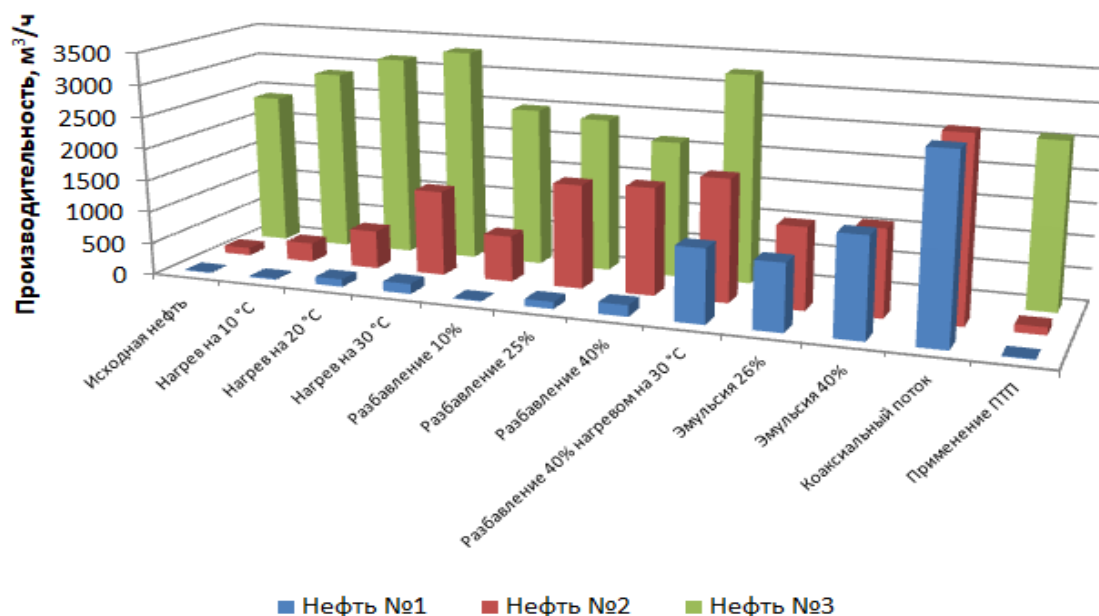
Рисунок 1 - Производительность нефтепровода при использовании различных методов транспортировки нефтей № 1, 2 и 3
