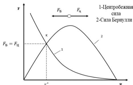
Рисунок 1 - Движущие силы гидроциклона
