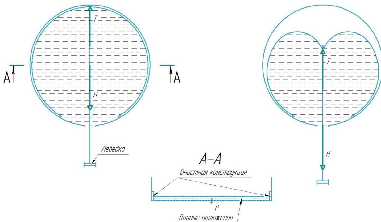
Рисунок 1 – Расчетная схема
