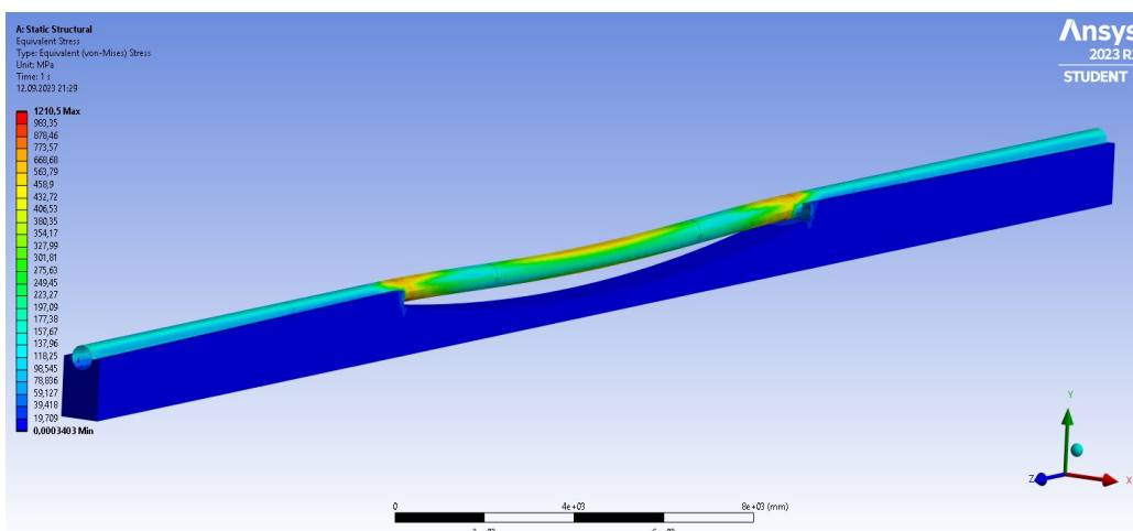
Рисунок 2 – График распределения напряжений до применения криогеля (max = 1210,5 МПа)
