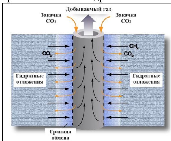
Рисунок 1 – Секвестрация \text{CO}_2 с обменом \text{CH}_4
