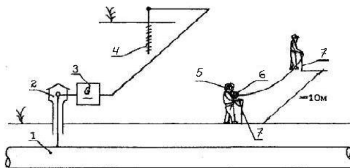
1 - труба, 2 - КИП, 3 - генератор звуковой частоты, 4 - временный заземлитель, 5 - головные телефоны, 6 - приемник ИПИ, 7 - стальные электроды
