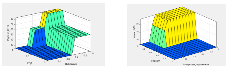
Рисунок 2 – Поверхность системы нечеткого вывода
