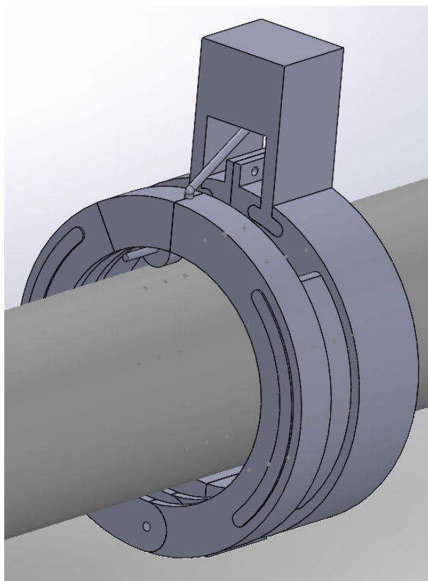
Рисунок 1 – Конструкция нанесения битумно-мастичного покрытия на наружную поверхность трубопровода
