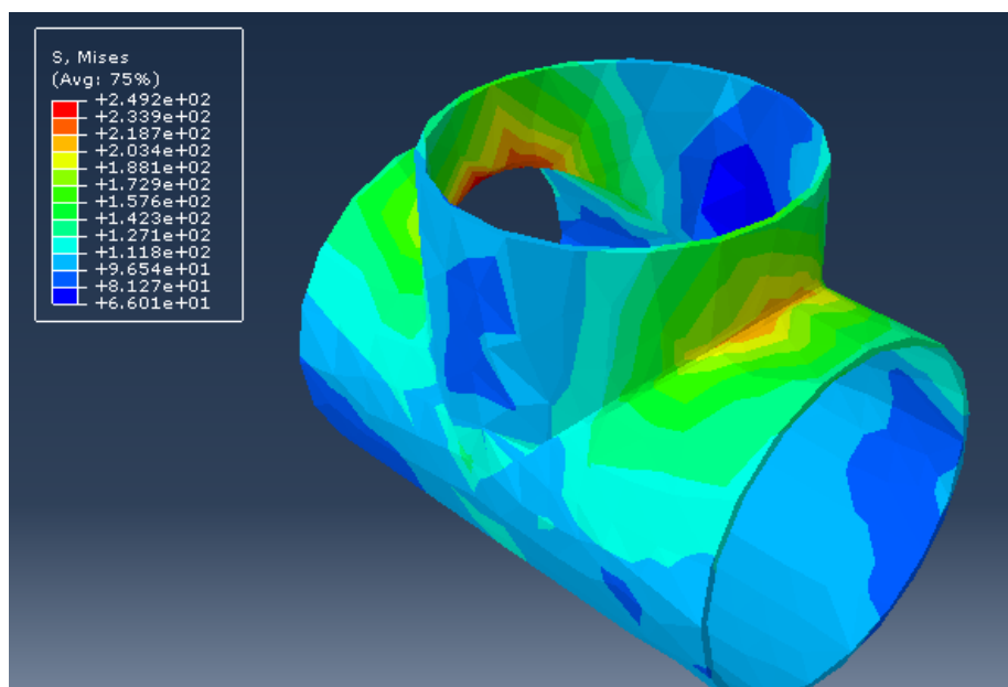
Рисунок 1 - Цифровая модель тройника в напряженном состоянии
