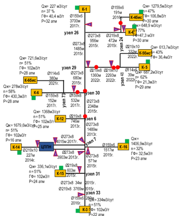
Рисунок 1 – Схема моделируемого месторождения
