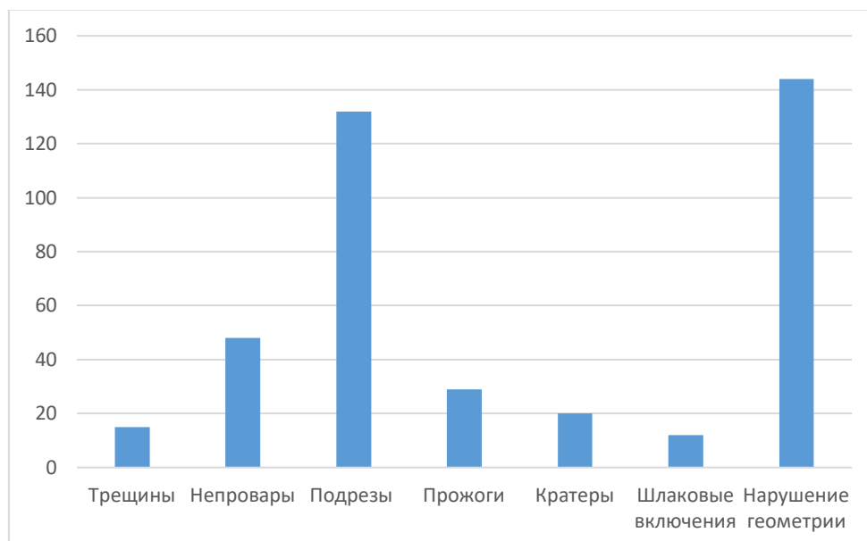
Рисунок 1 – Распределение дефектов в сварных соединениях
