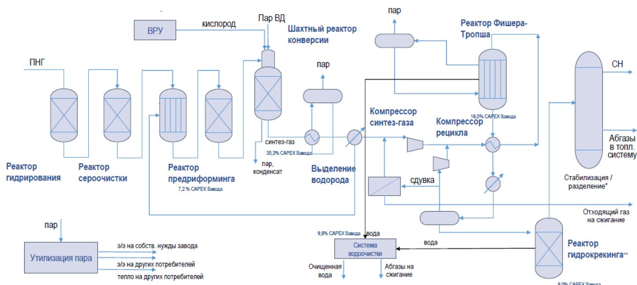
Рисунок 1 – Технологическая блок-схема процесса
