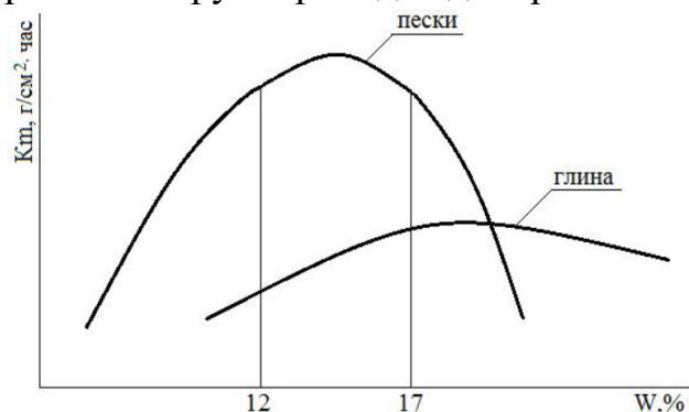
Рисунок 2 – Зависимость установившейся скорости коррозии от влажности и типа грунта
