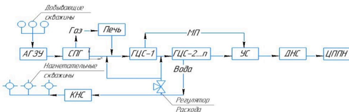
Рисунок 1 – Принципиальная схема автоматизированной установки
