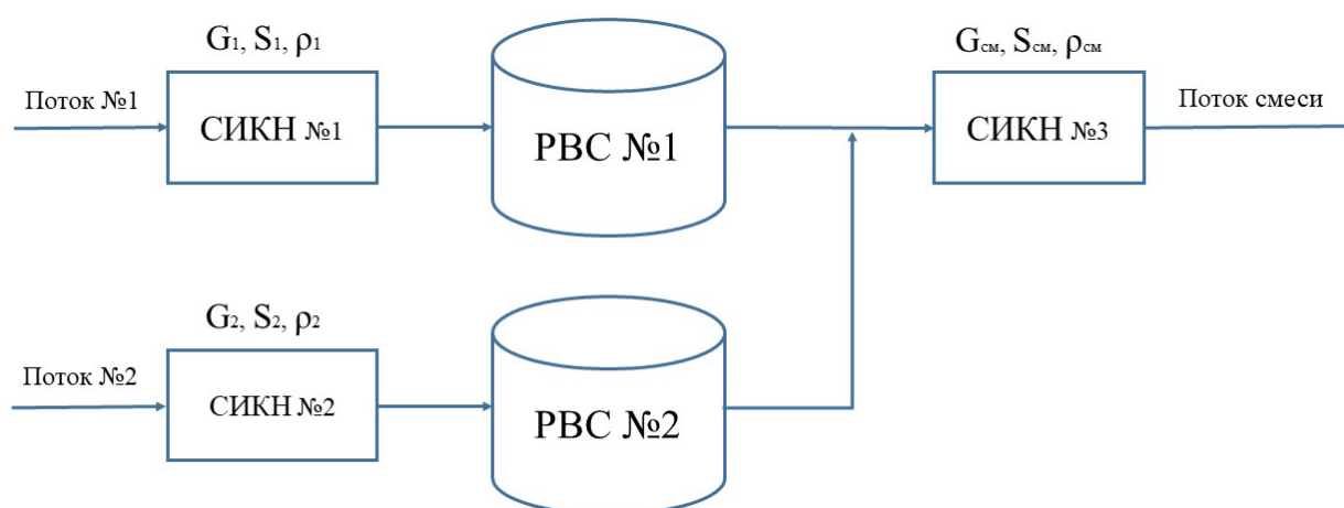
Рисунок 2 – Схема смешения потоков нефти
