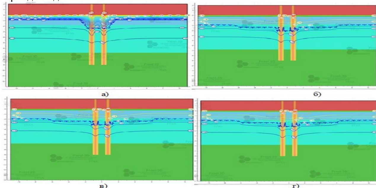
Рисунок 1 – Результат расчета теплового поля в виде изолиний температуры в поперечном сечении опорной зоны моделирования на всю глубину залегания
