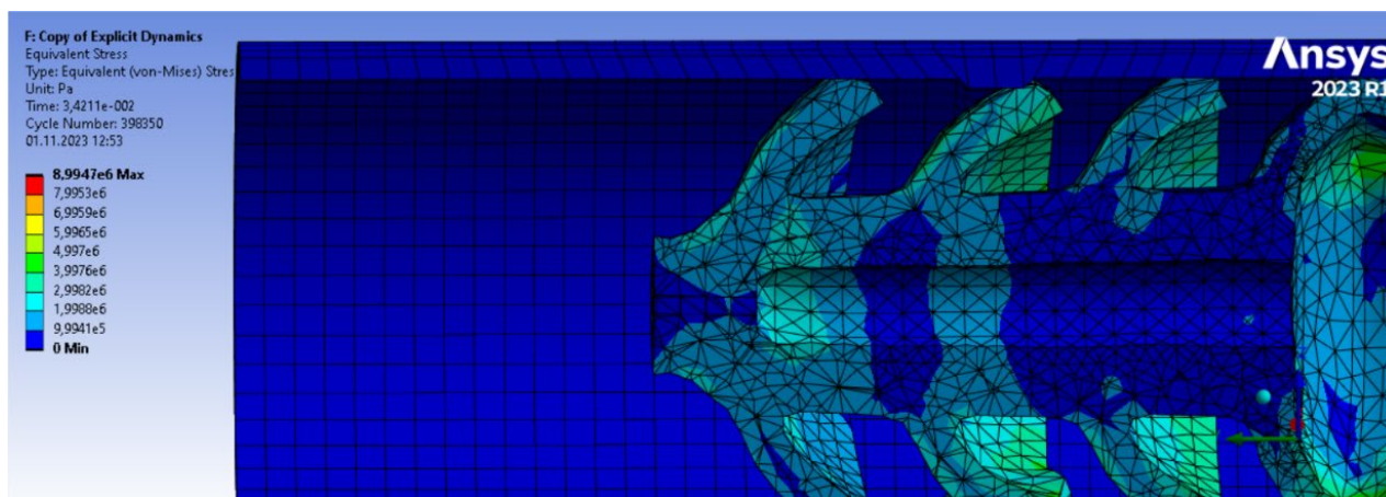
Рисунок 1 – Моделирование прохождения внутритрубным снарядом локального места сужения 85% от наружного диаметра трубопровода
