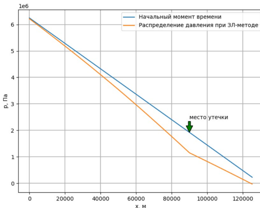
Рисунок 1 – Визуализация моделирования нестационарного процесса на магистральном нефтепроводе в программной комплексе
