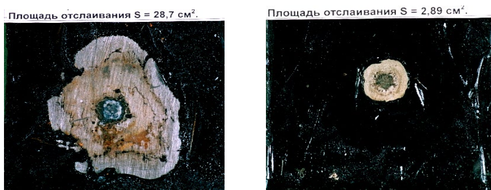
Рисунок 2 – Результаты испытаний на стойкость к катодному отслаиванию
