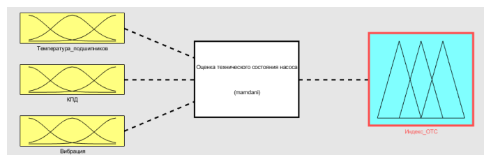
Рисунок 1 - Структурная схема оценки технического состояния МНА
