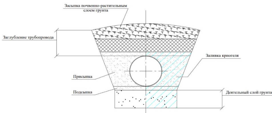
Рисунок 1 – Подземная прокладка магистрального ТП с использованием криогеля
