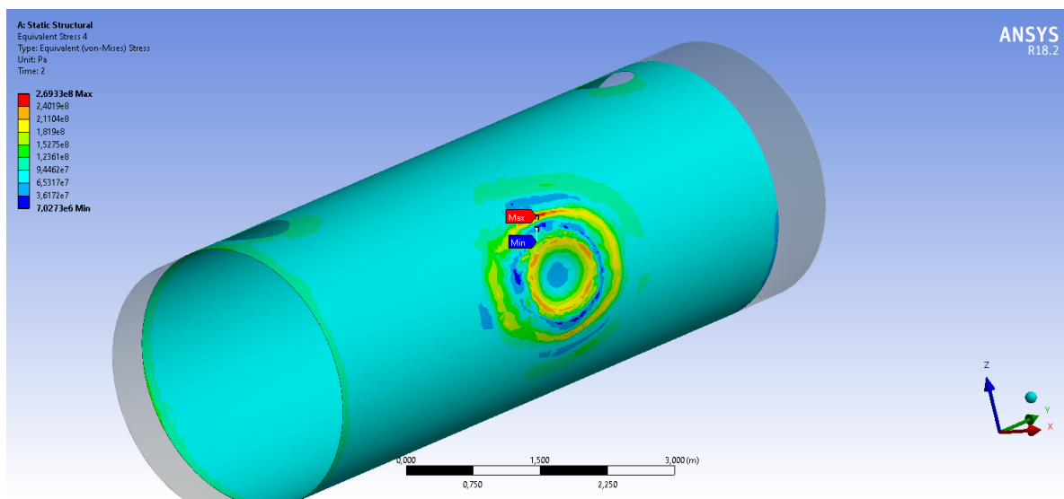
Рисунок 2 – Остаточные напряжения при вмятине с глубиной 15 см
