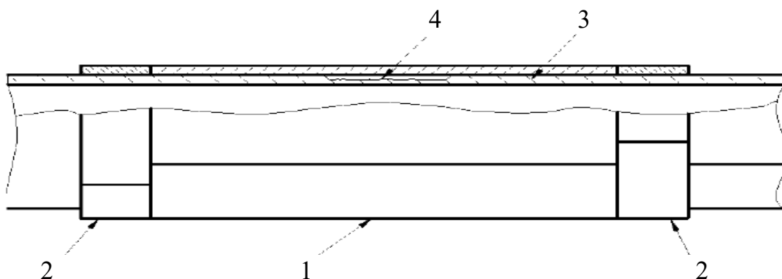
1 – центральное кольцо; 2 – технологическое кольцо; 3 – труба; 4 – дефект Рисунок 1 – Муфта обжимная приварная с технологическими кольцами (тип П2)
