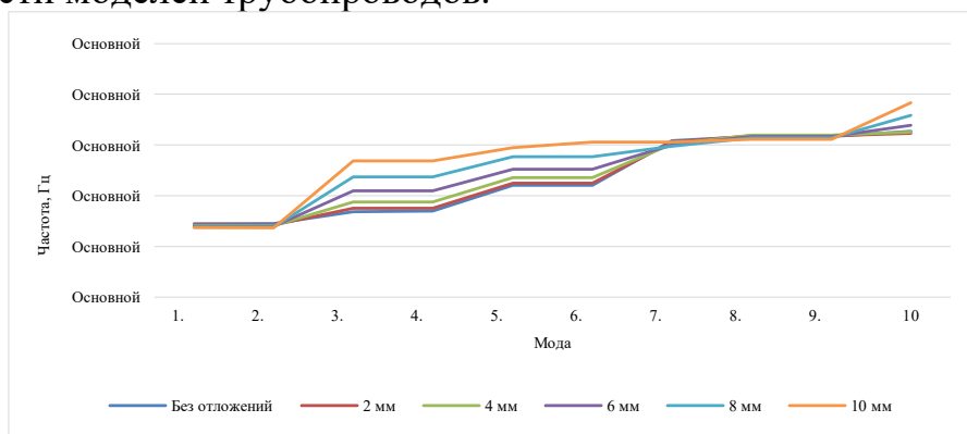
Рисунок 1 – Анализ собственных частот трубопровода
