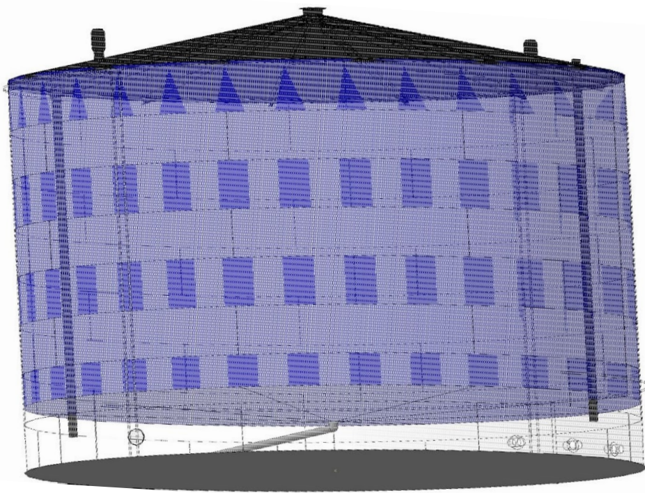
Рисунок 2 – Вид резервуара с мягкой оболочкой с обратной стороны *стенка резервуара и мягкая оболочка для наглядности показаны прозрачными
