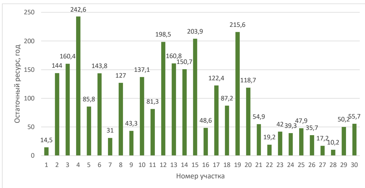
Рисунок 2 – Диаграмма полученных результатов остаточного ресурса для различных участков трубопровода
