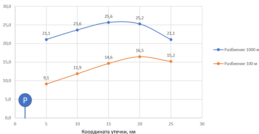
Рисунок 2 – Влияние расположения утечки на величину импульса в процентах от давления на конце участка
