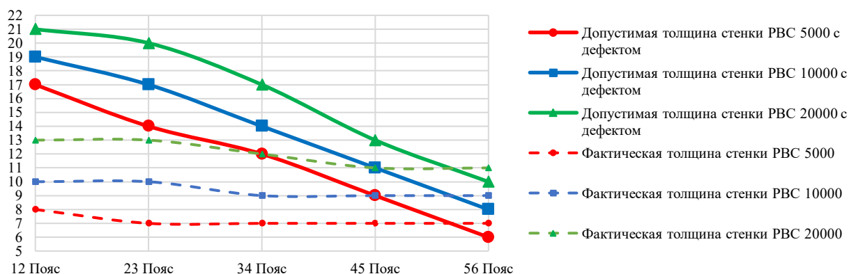
Рисунок 2 – Дефект с высотой 3000 мм
