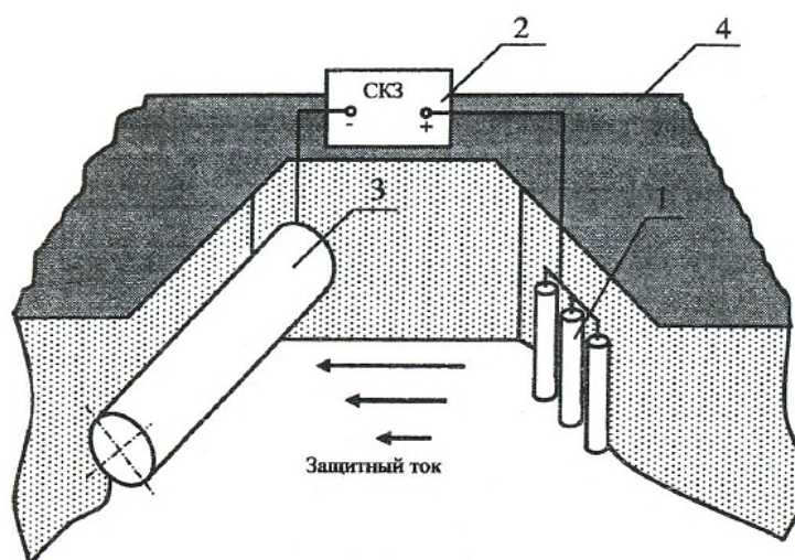
1 – анодное заземление; 2 – станция катодной защиты (источник тока); 3 – трубопровод; 4 - грунт
