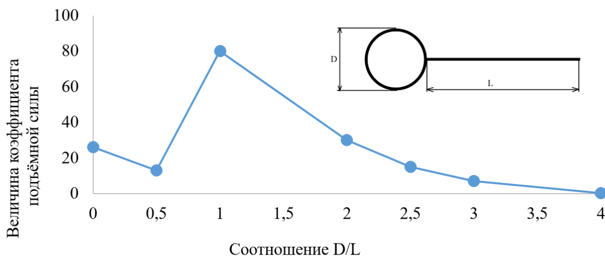
Рисунок 1 – Зависимость коэффициента подъемной силы от длины «сплиттера»
