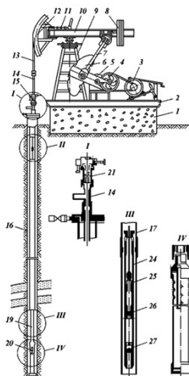
Рисунок 1 – Пример схемы глубинной скважинной установки [3]
