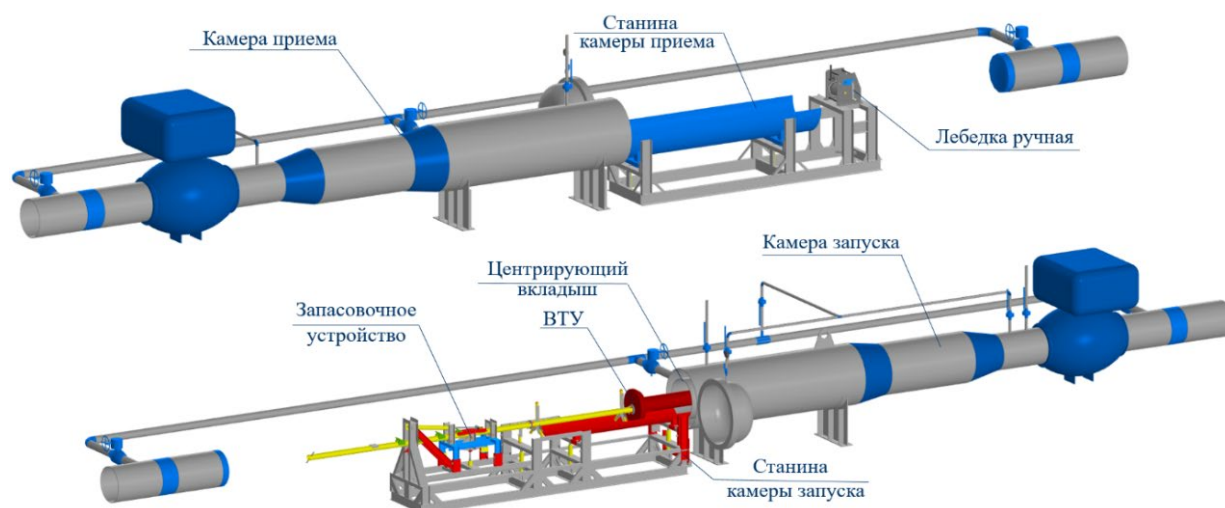
Рисунок 1 – Универсальный мобильный комплекс (на примере DN 700)
