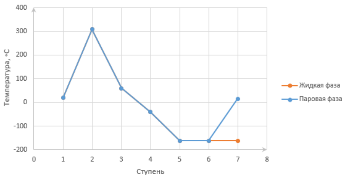
Рисунок 1 – Изменение температуры природного газа на разных ступенях технологической схемы сжижения
