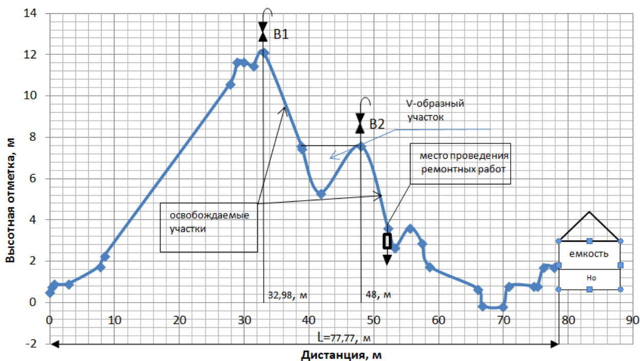
Рисунок 1 – Профиль БИГ для угла наклона 23 градуса
