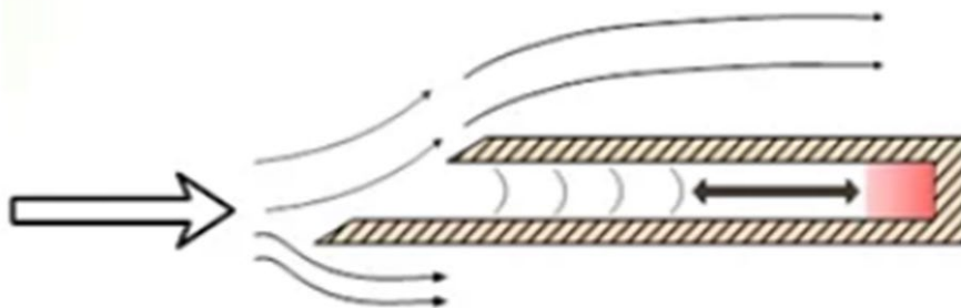
Рисунок 1 – Возникновение эффекта Гартмана-Шпренгера
