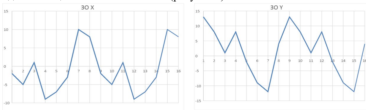
Рисунок 1 - Биение измерительной поверхности на радиальной опоре со стороны свободного конца
