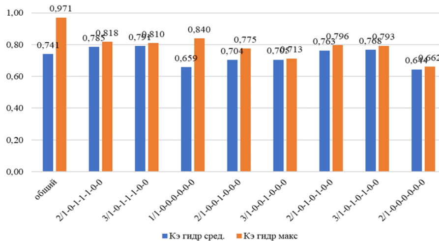
Рисунок 1 – K_{\text{гидр}} – инструмент анализа эффективности линейной части ТУ МН при различных технологических режимах перекачки
