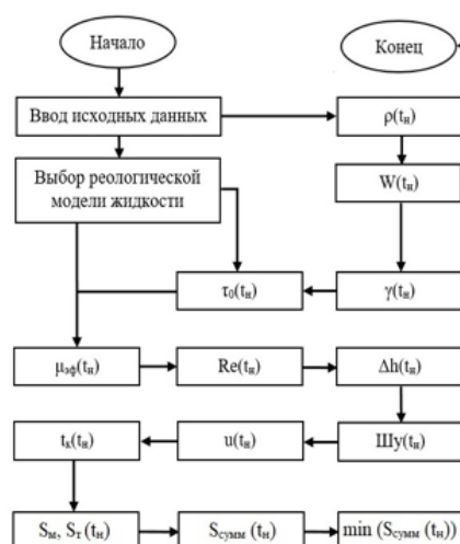
Рисунок 1 - Алгоритм расчета оптимальных параметров «горячей» перекачки ВВН с учетом минимальных эксплуатационных затрат
