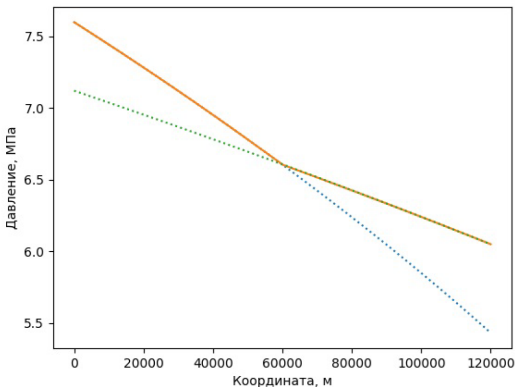
Рисунок 1 – Пример распределения давления, получаемого при моделировании
