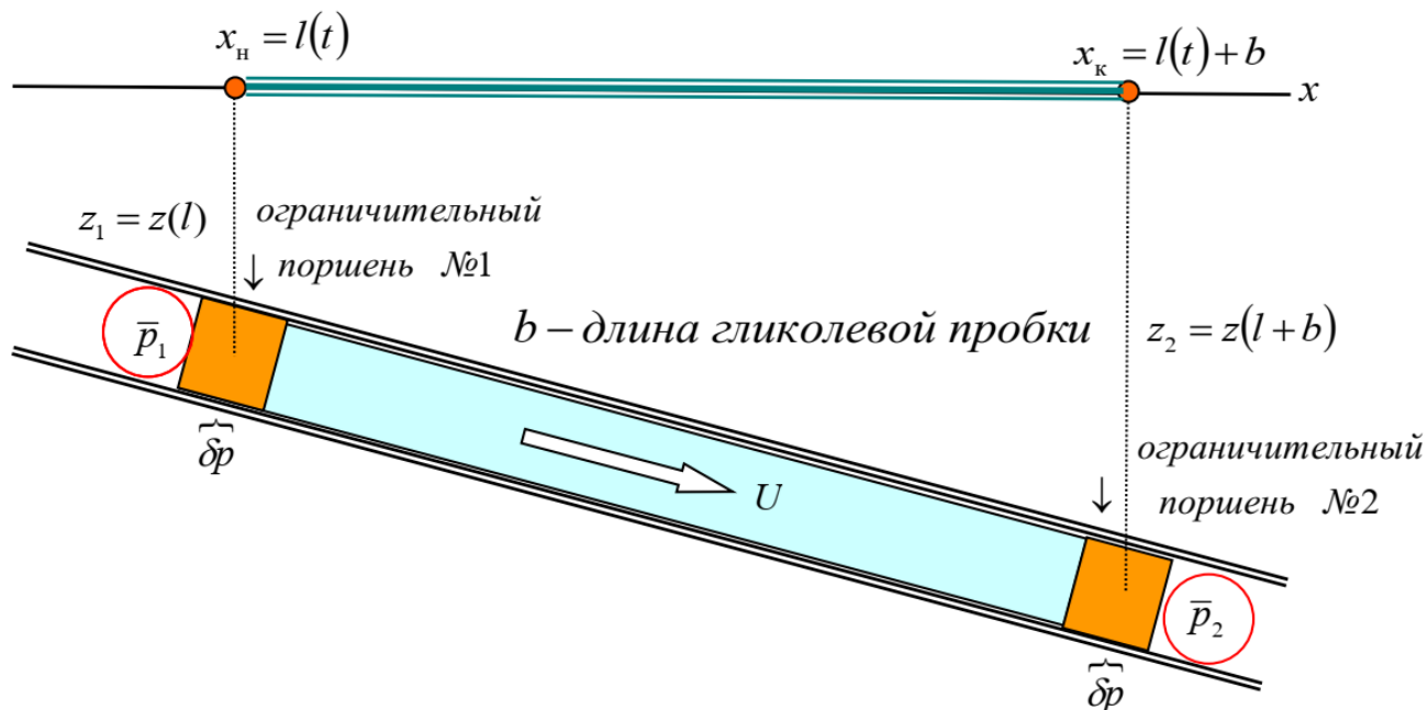
Рисунок 1 - Схема жидкостной пробки в трубопроводе
