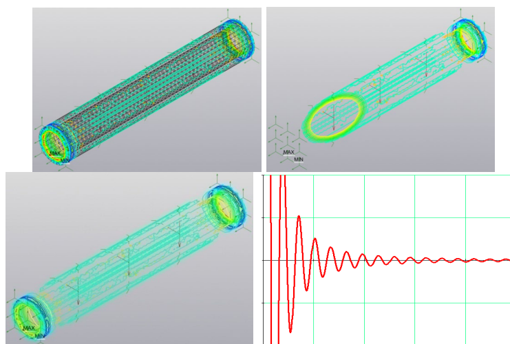
Рисунок 1 – Результаты моделирования распространения линейно направленных ультразвуковых волн в моделируемом участке полиэтиленового трубопровода
