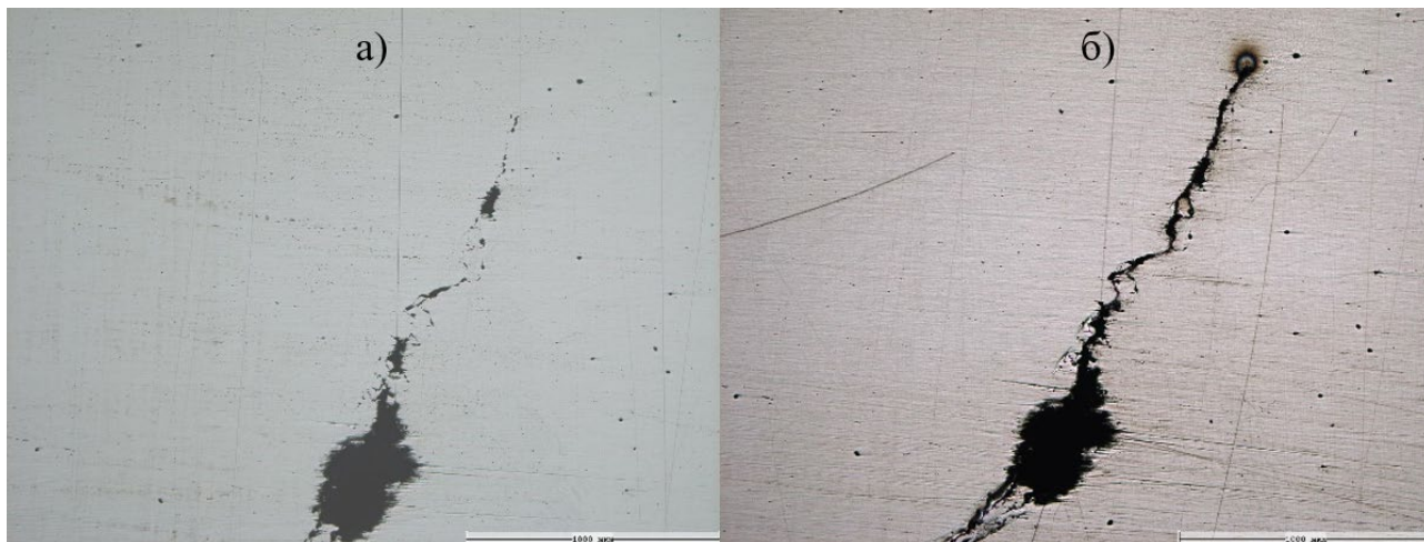
Рисунок 2 – Изображение трещины: а) исходное состояние вершины микротрещины при 50-кратном увеличении; б) изображение конца после МИО-20 кДж при 50-кратном увеличении
