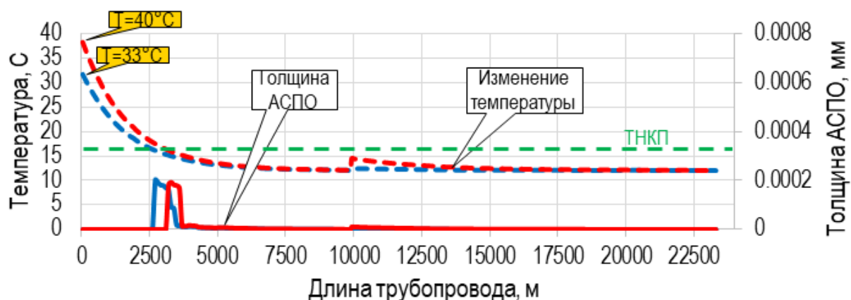
Рисунок 1 – Результат гидравлического расчета трубопровода для наглядного определения участков образований АСПО в летний период
