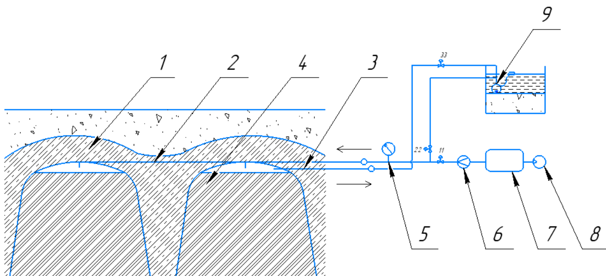
Рисунок 1 – Функциональная схема системы управления с помощью воздуха
