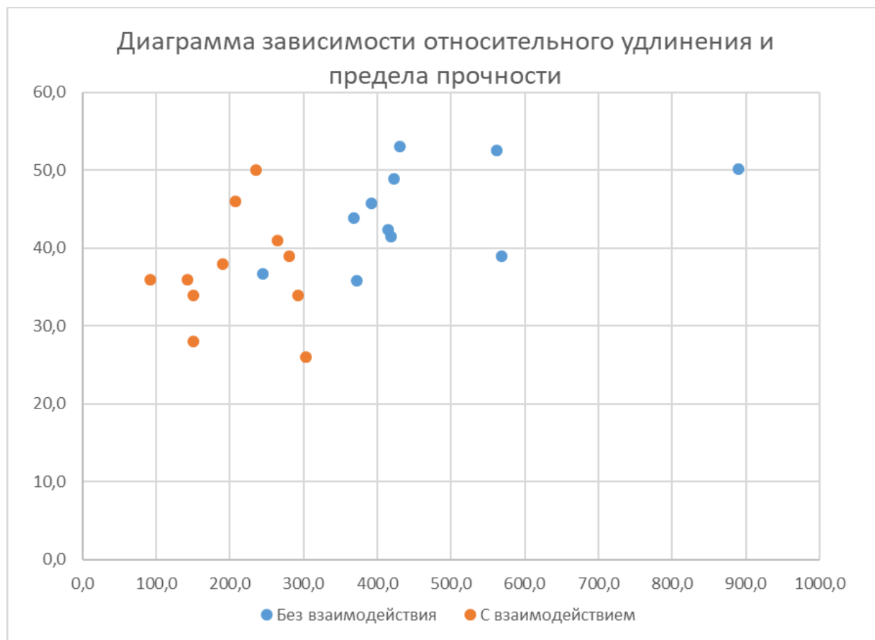
Рисунок 4 - Диаграмма зависимости относительного удлинения и предела прочности
