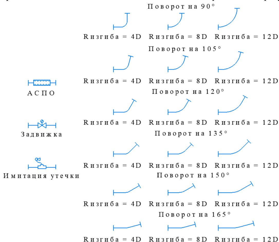
Рисунок 2 – Принципиальные схемы основных сменных секций
