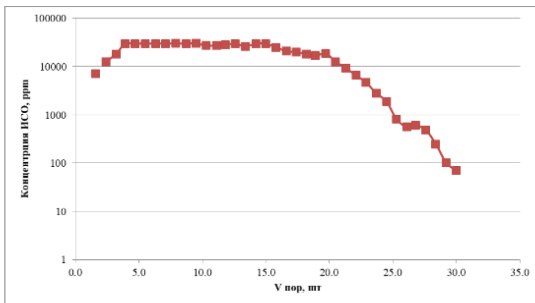
Рисунок 3.18 – Остаточное содержание реагента в пробах на выходе из колонки
