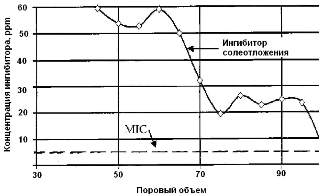
Рисунок 1.5 – Вынос ингибитора солеотложения при прокачке воды [52]
