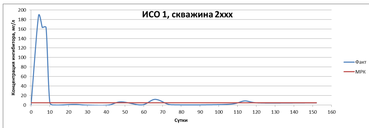
Рисунок 4.5 – Вынос ИСО 1 после задавки 2ххх
