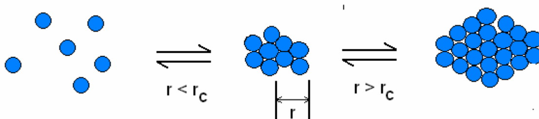
Рисунок 1.15 – Агрегация молекулярных кластеров, ведущих к зарождению кристалла
