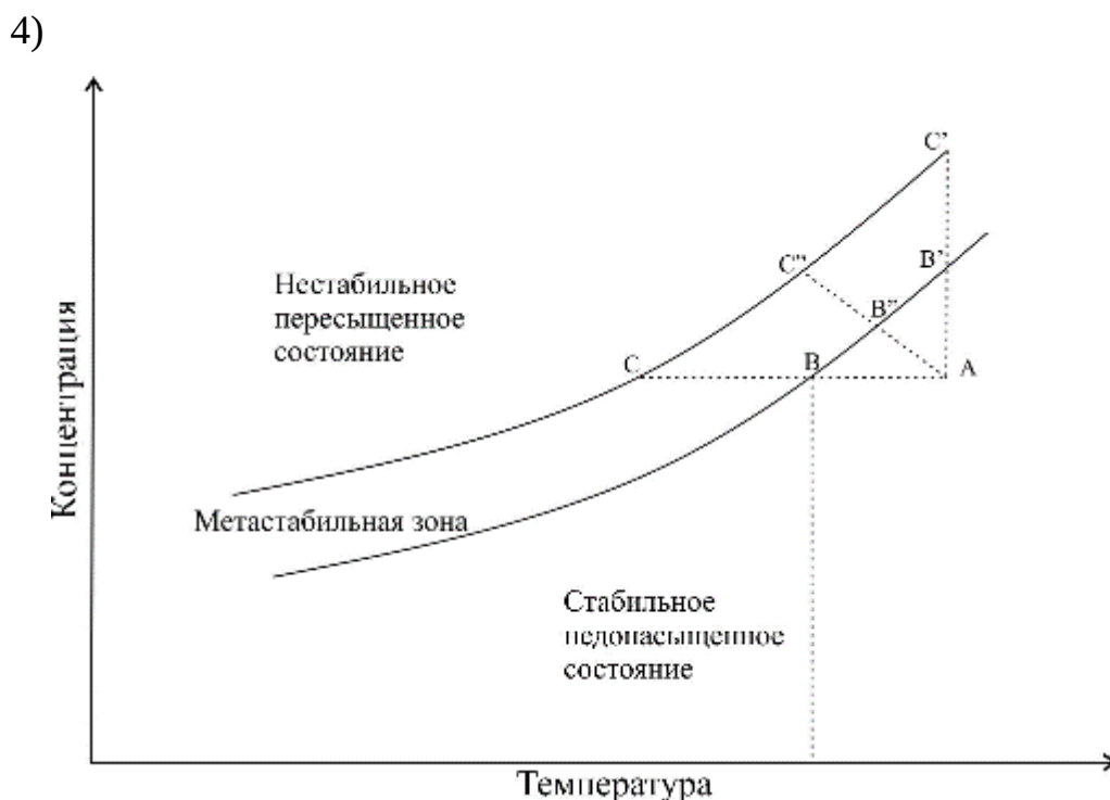
Рисунок 1.14 – Диаграмма фазового состояния раствора хлорида натрия
