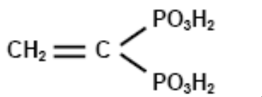
Рисунок 1.7 – Структурная формула ВДФК
