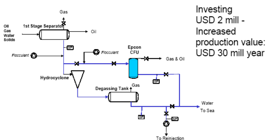
Рисунок 1.1 – Принципиальная схема водоподготовки Epcor CFU Technology путем очистки пластовой воды флокулянтами перед сбросом ее в море
