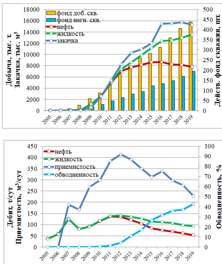
Рисунок 1.25 – Динамика основных показателей разработки рассматриваемого месторождения
