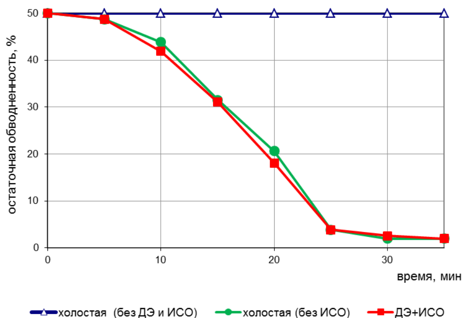
Рисунок 3.23 - Динамика отстоя эмульсий (обводн. 50 %) на основе нефти месторождения NN с добавкой реагента в условиях УПН-1 по содержанию остаточной воды
