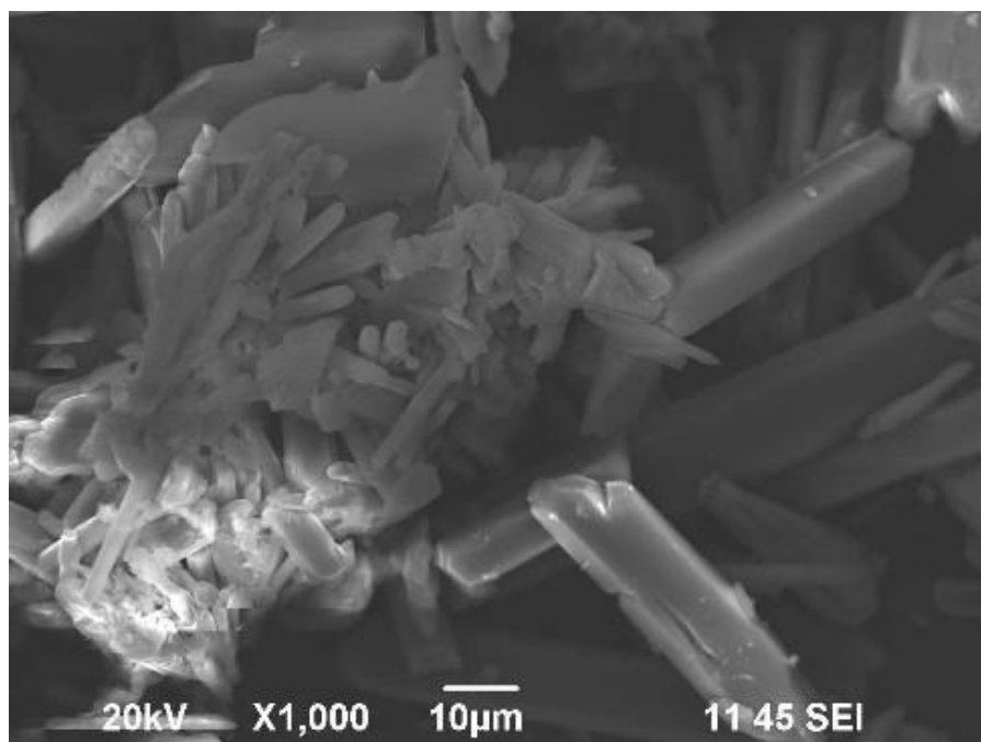
Рисунок 3.9 – Кристаллы гипса в холостом эксперименте (без обработки реагента)
