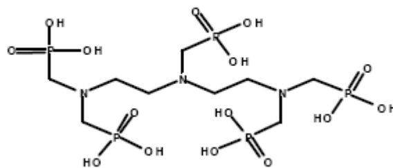
Этилентриамин пента (метиленфосфоновая кислота)
