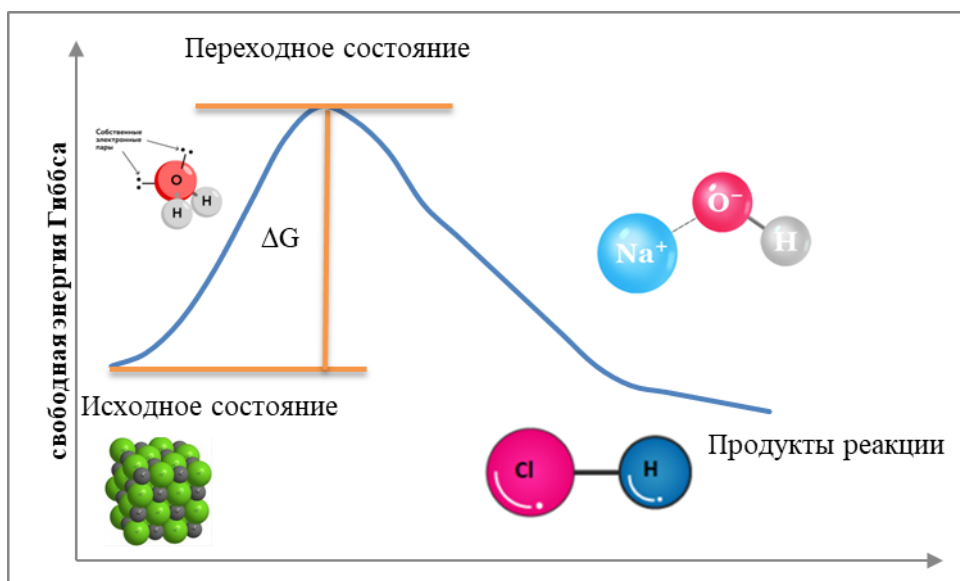
Рисунок 1.12 - Кривая потенциальной энергии растворения NaCl
